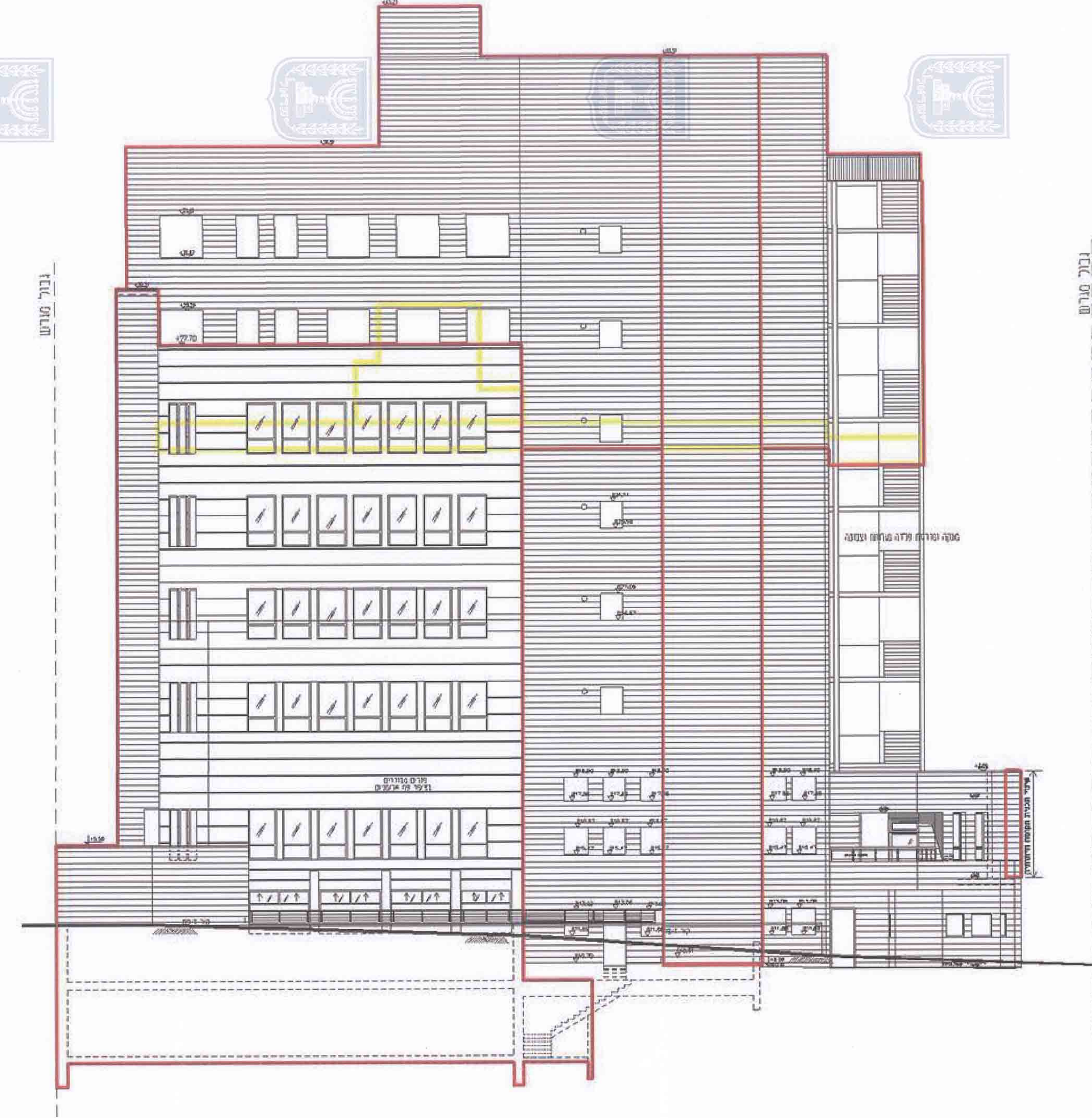
חזית מזרחית קנ"מ 1:100 ±0.00 = 810.43
