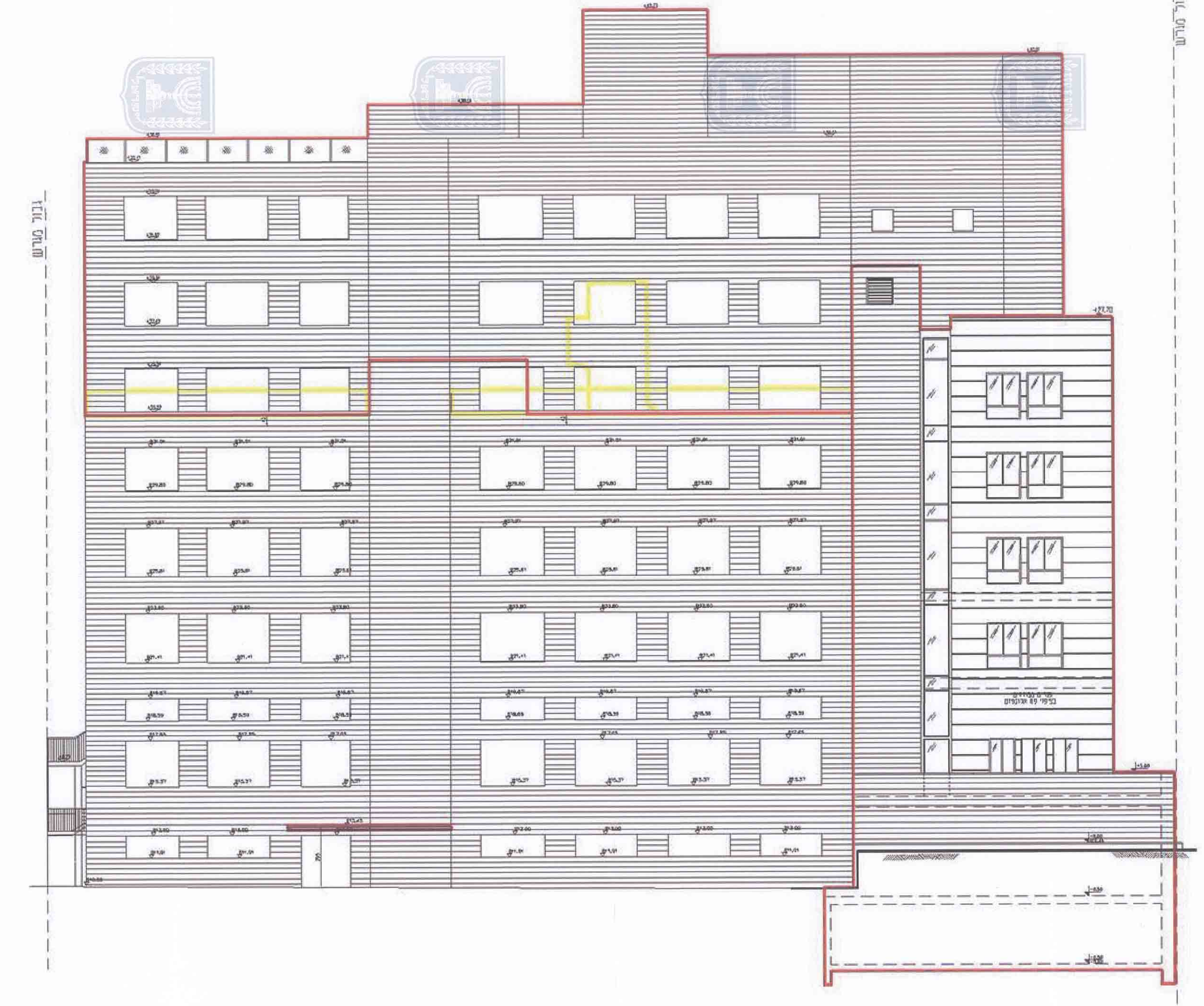
חזית דרומית קנ"מ 1:100 ±0.00 = 810.43
