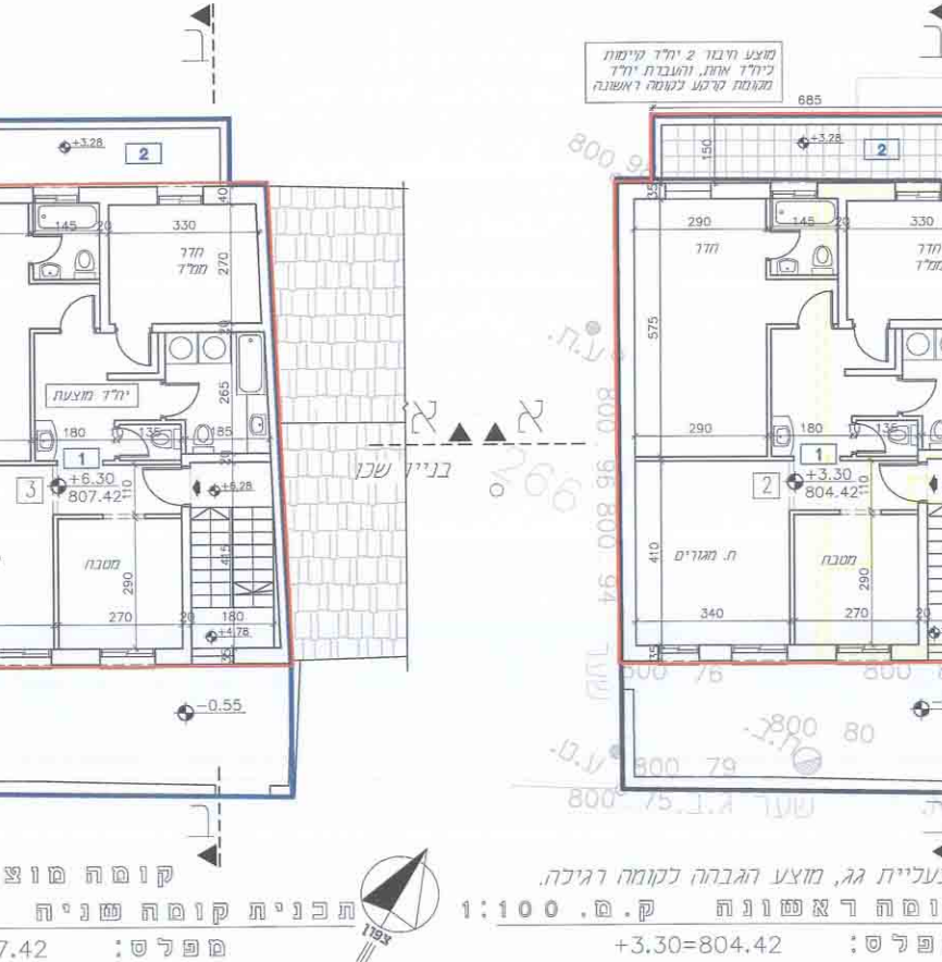
תכנית קו הממשל 1:100
