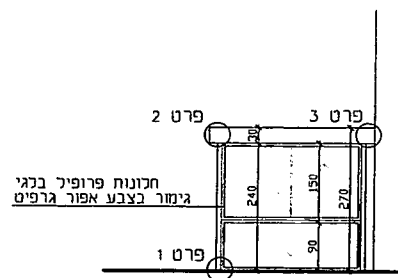
חזית דרומית ק.מ. 1:100
