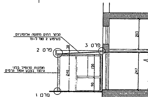
חזית מזרחית ק.מ. 1:100
