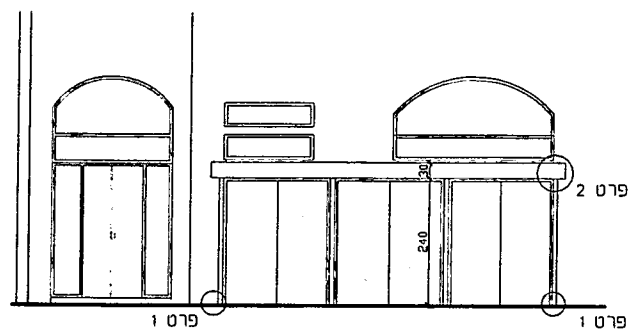
חזית מערבית ק.מ. 1:100
