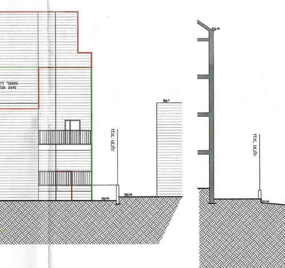
1:100 .ב.פ. חזית צפונית
