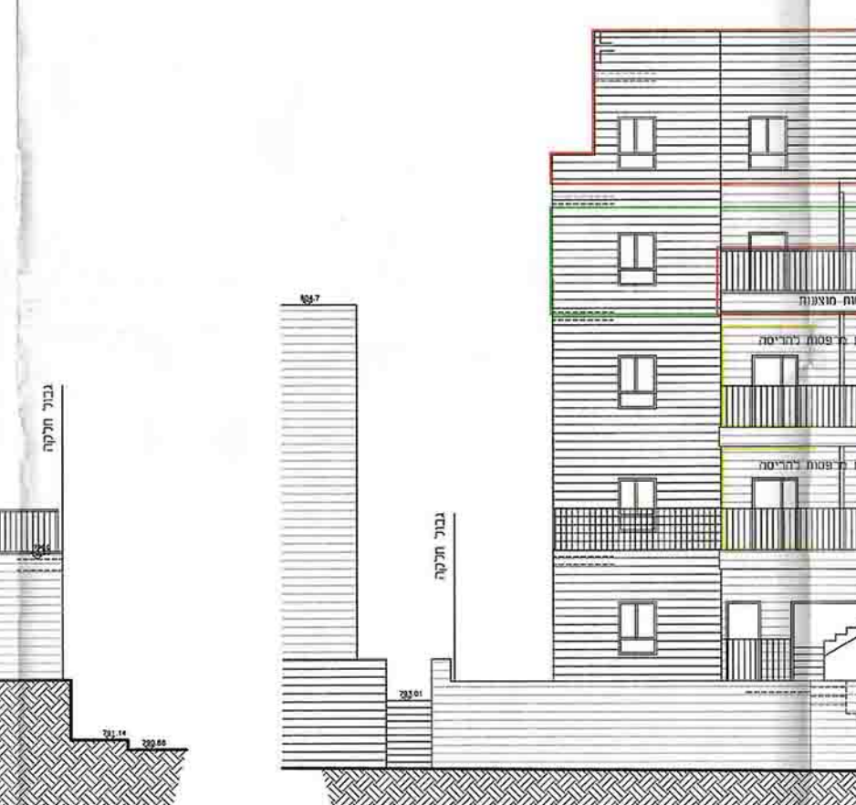
1:100 .ב.פ. חזית מזרחית
