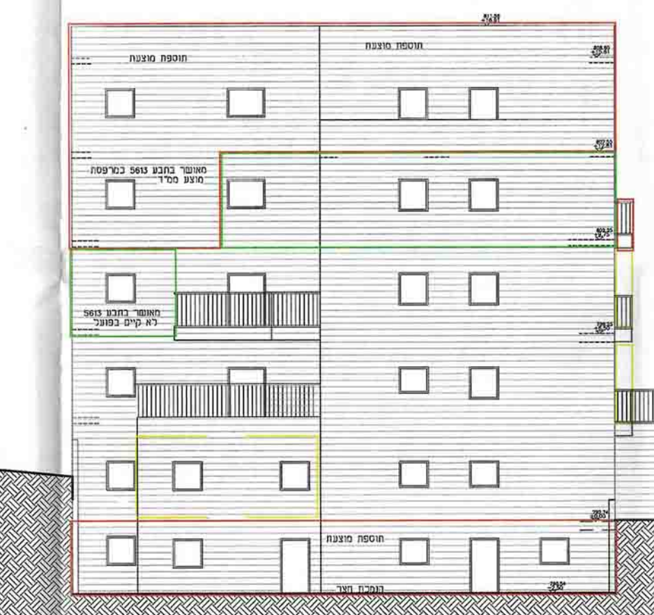
1:100 .ב.פ. חזית מערבית
