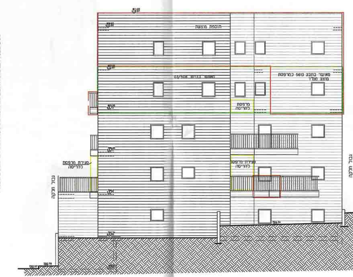
1:100 .ב.פ. חזית דרום
