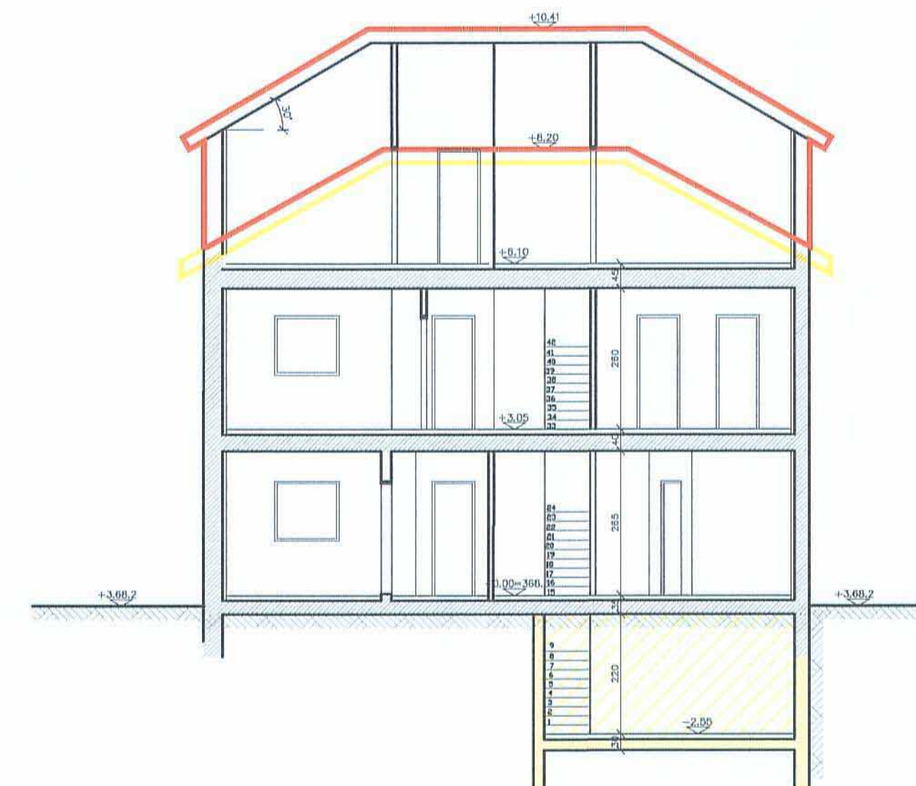
חתך א'-א' קני"מ: 1:100
