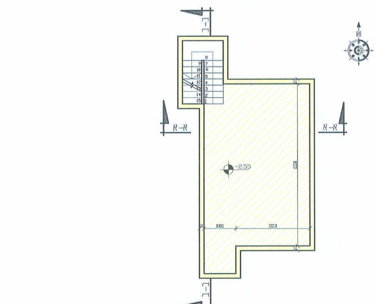
תכנית קומת מרתף-לביטול קני"מ: 1:100
