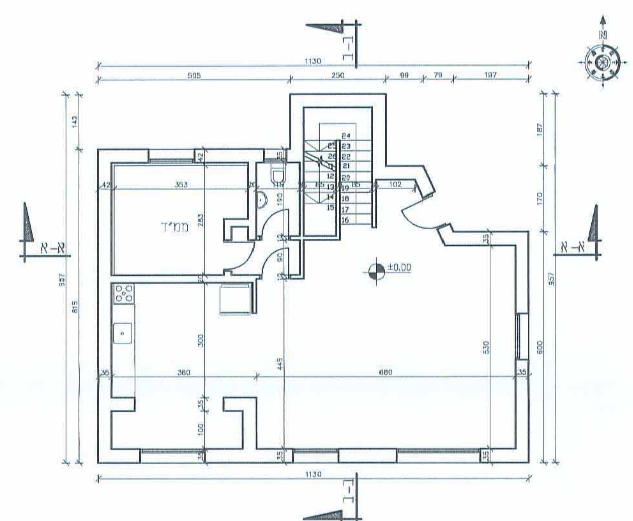
תכנית קומת כניסה קני"מ: 1:100
