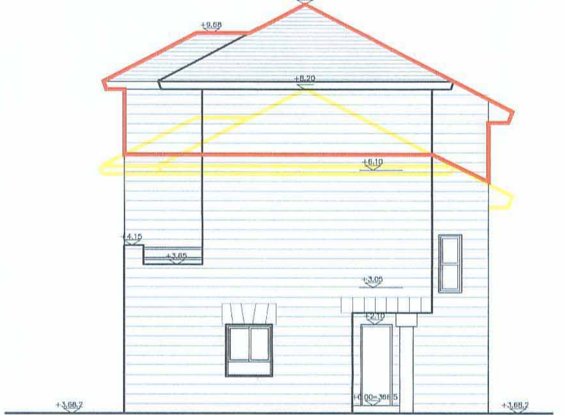
חזית מזרחית קני"מ: 1:100
