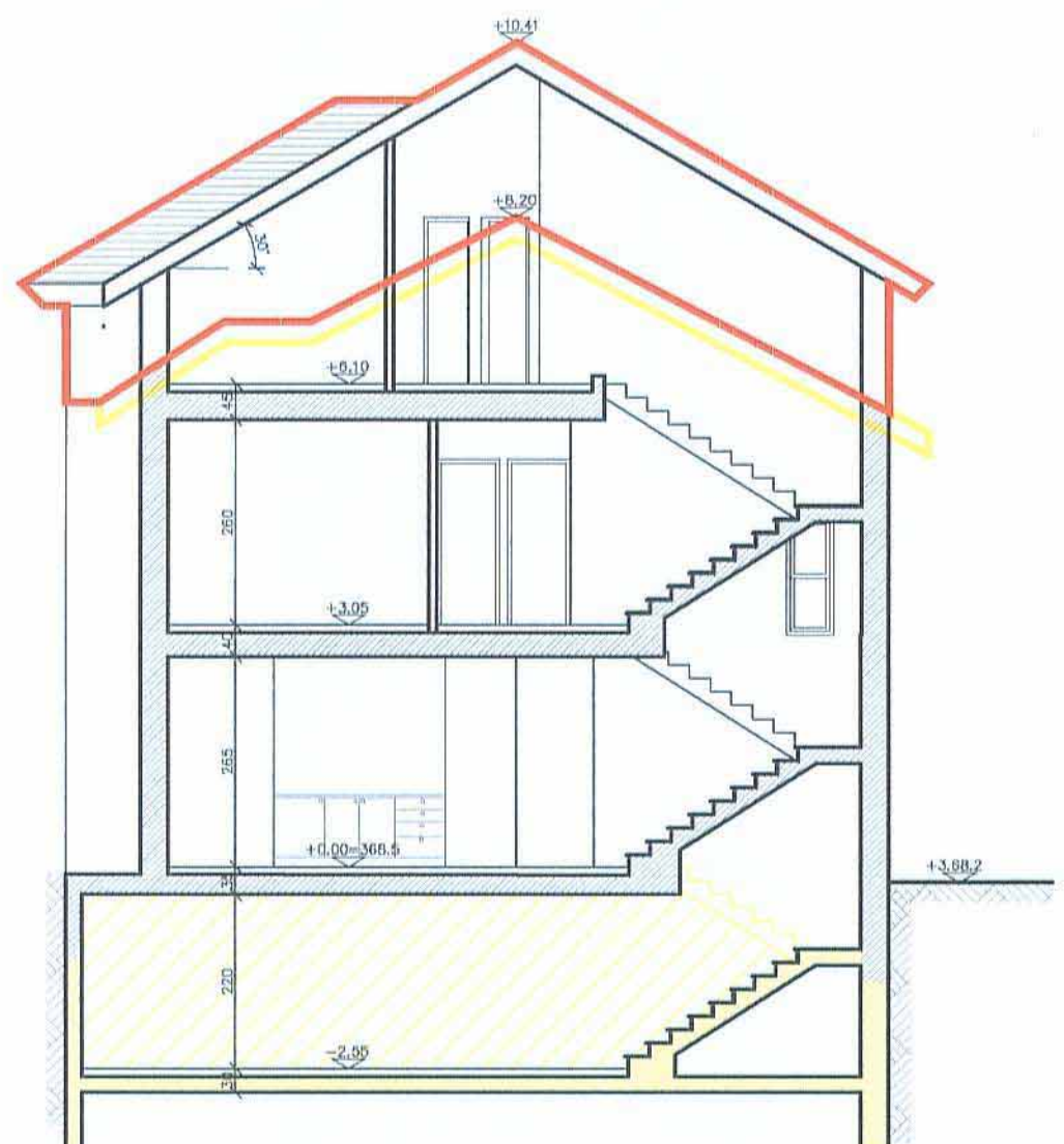
חתך ב-ב קני"מ: 1:100
