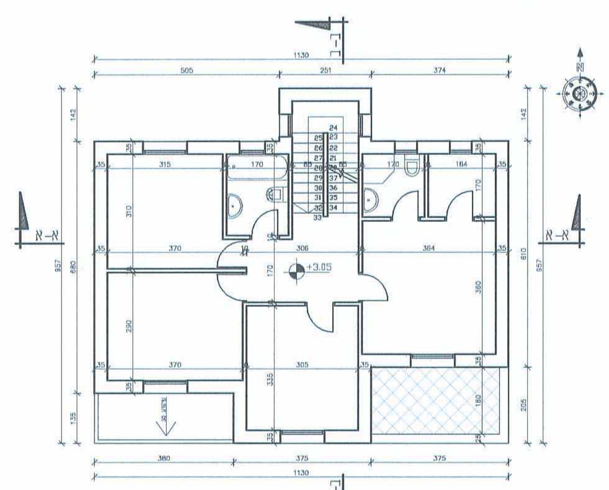
תכנית קומה א' קני"מ: 1:100
