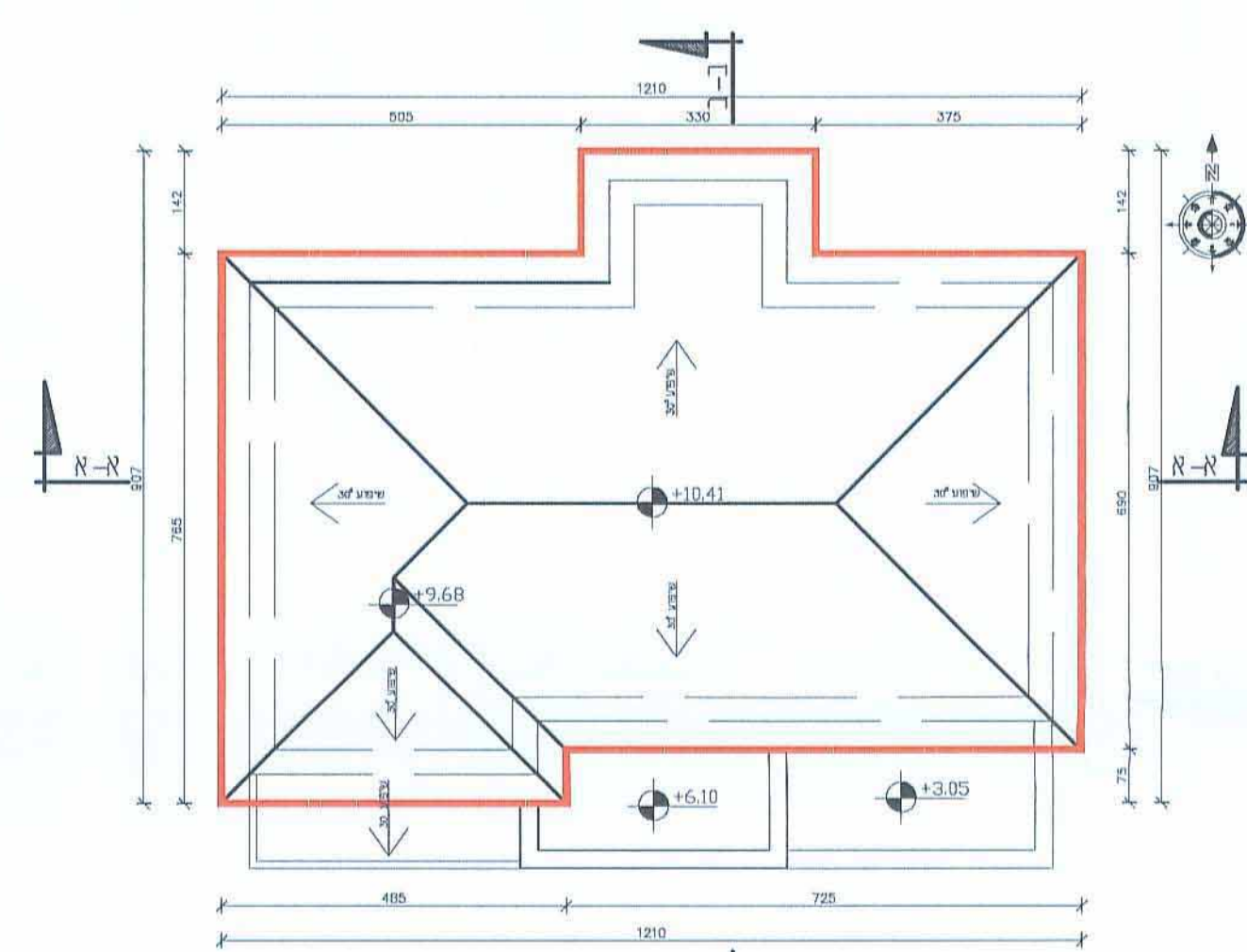
תכנית גגות קני"מ: 1:100
