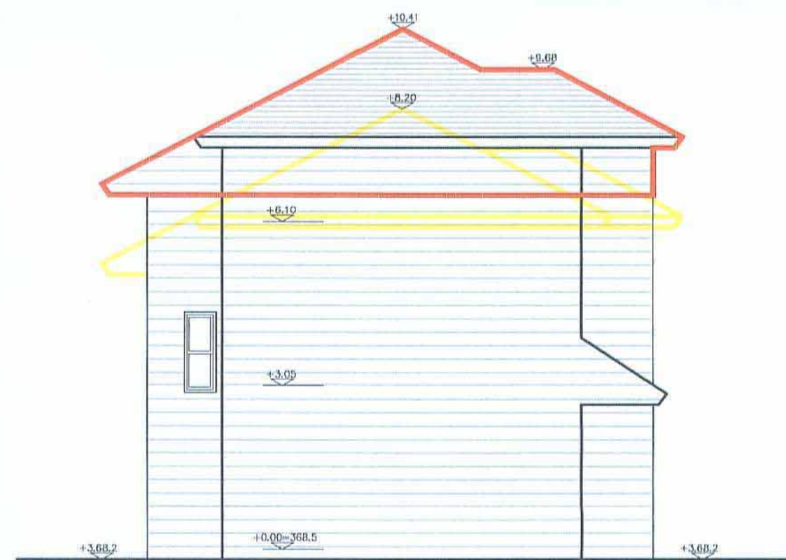
חזית מערבית קני"מ: 1:100
