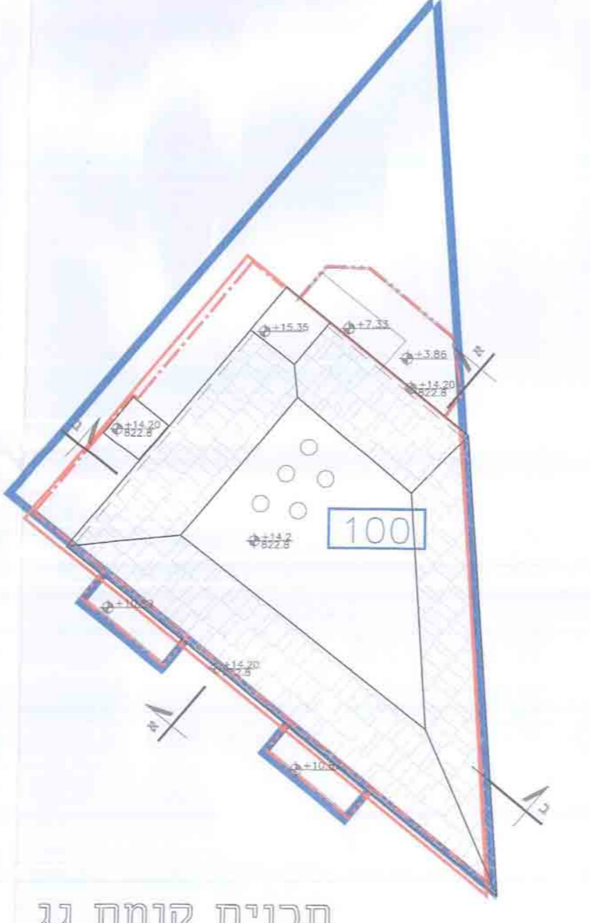
תכנית קומת גג במפרט +14.20 = 822.8 קנ"מ 1:100
