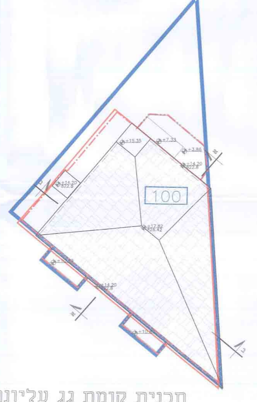
תכנית קומת גג עליונה קנ"מ 1:100
