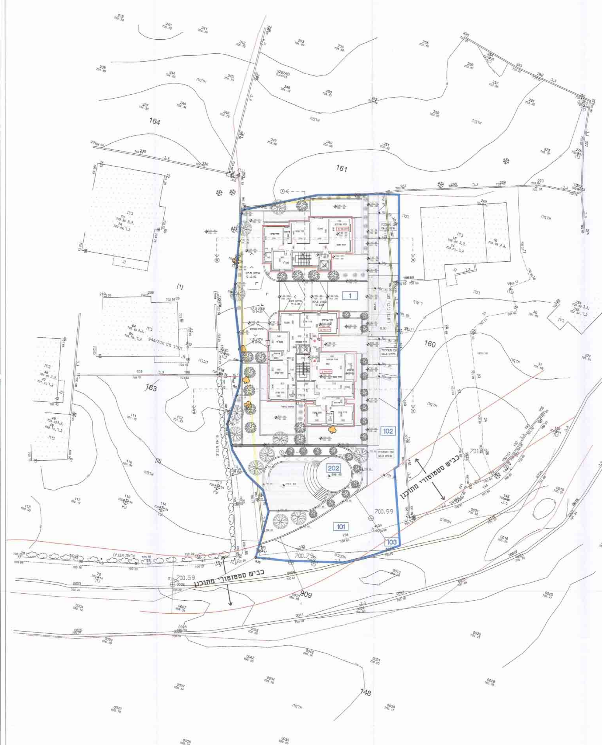
תכנית קומת פיתוח+ארקע מפלס 00 ± (701.80) קנ"מ 1:200
