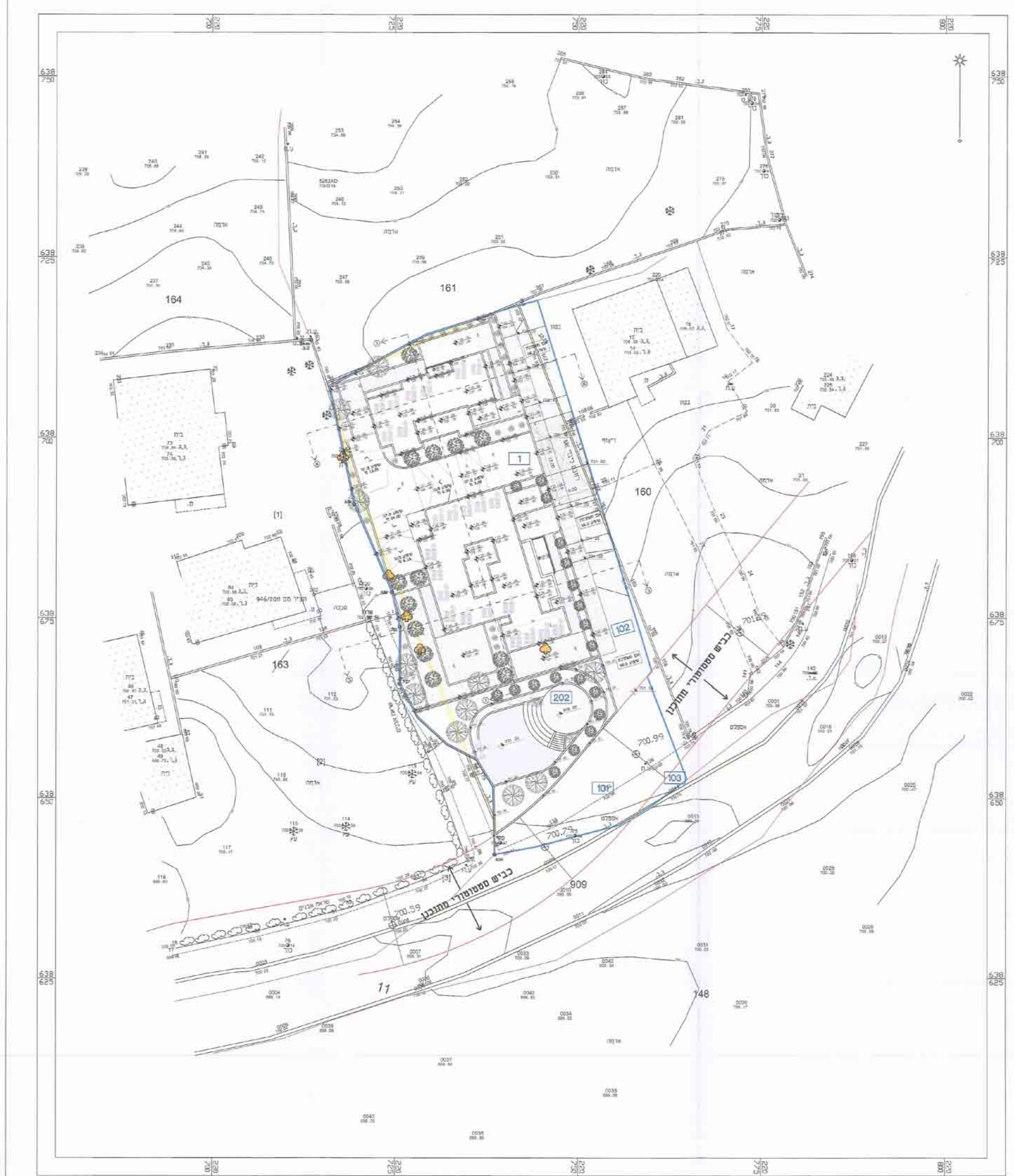
תוכנית פיתוח קנ"מ 1:250
