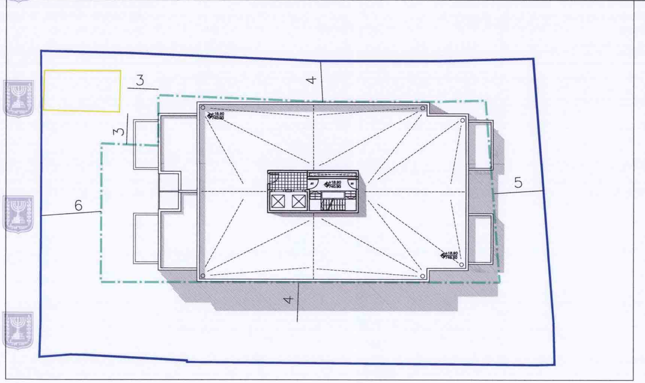
תכנית גג
