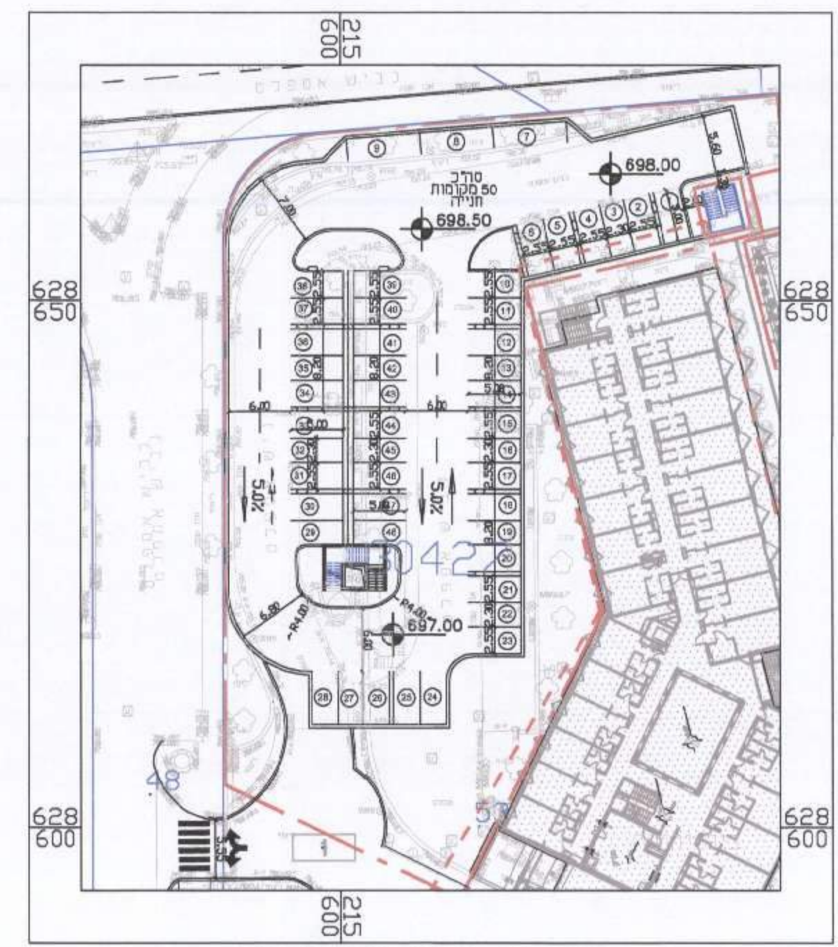
מפלס חניה טיפוסי
