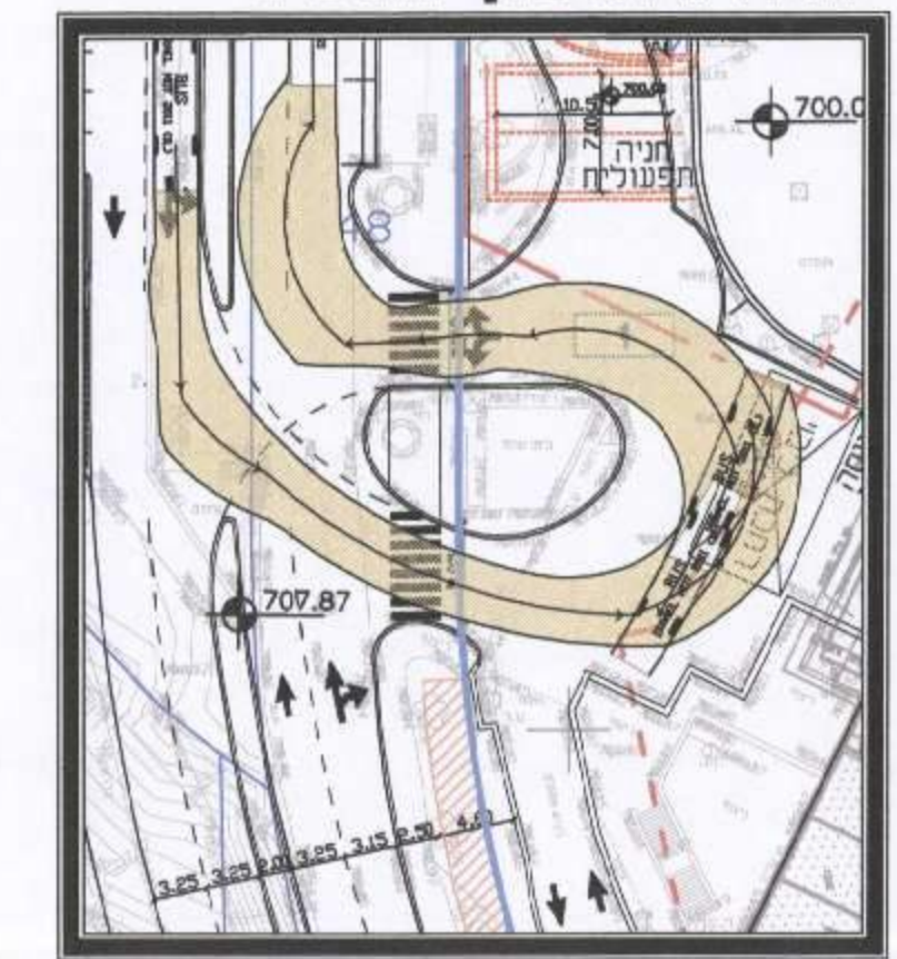
תמרון אוטובוס הורדה ואיסוף נוסעים
