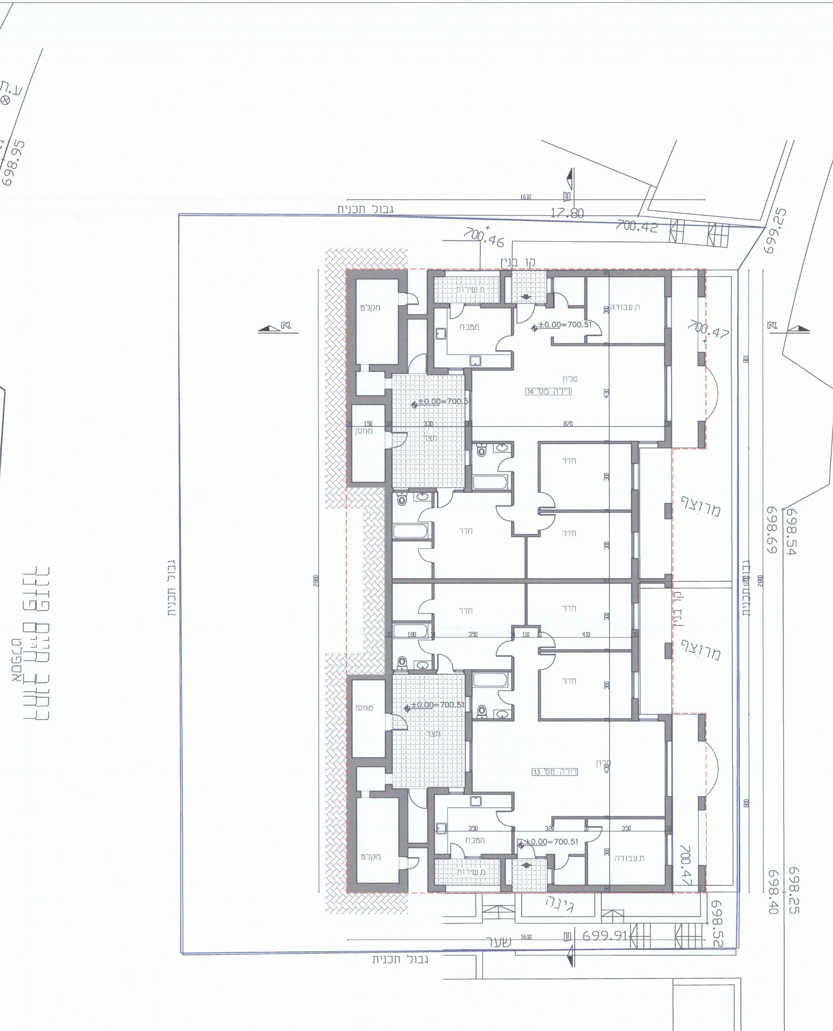
תכנית קומת קרקע +0.00=700.51 קנ"מ 1:100
