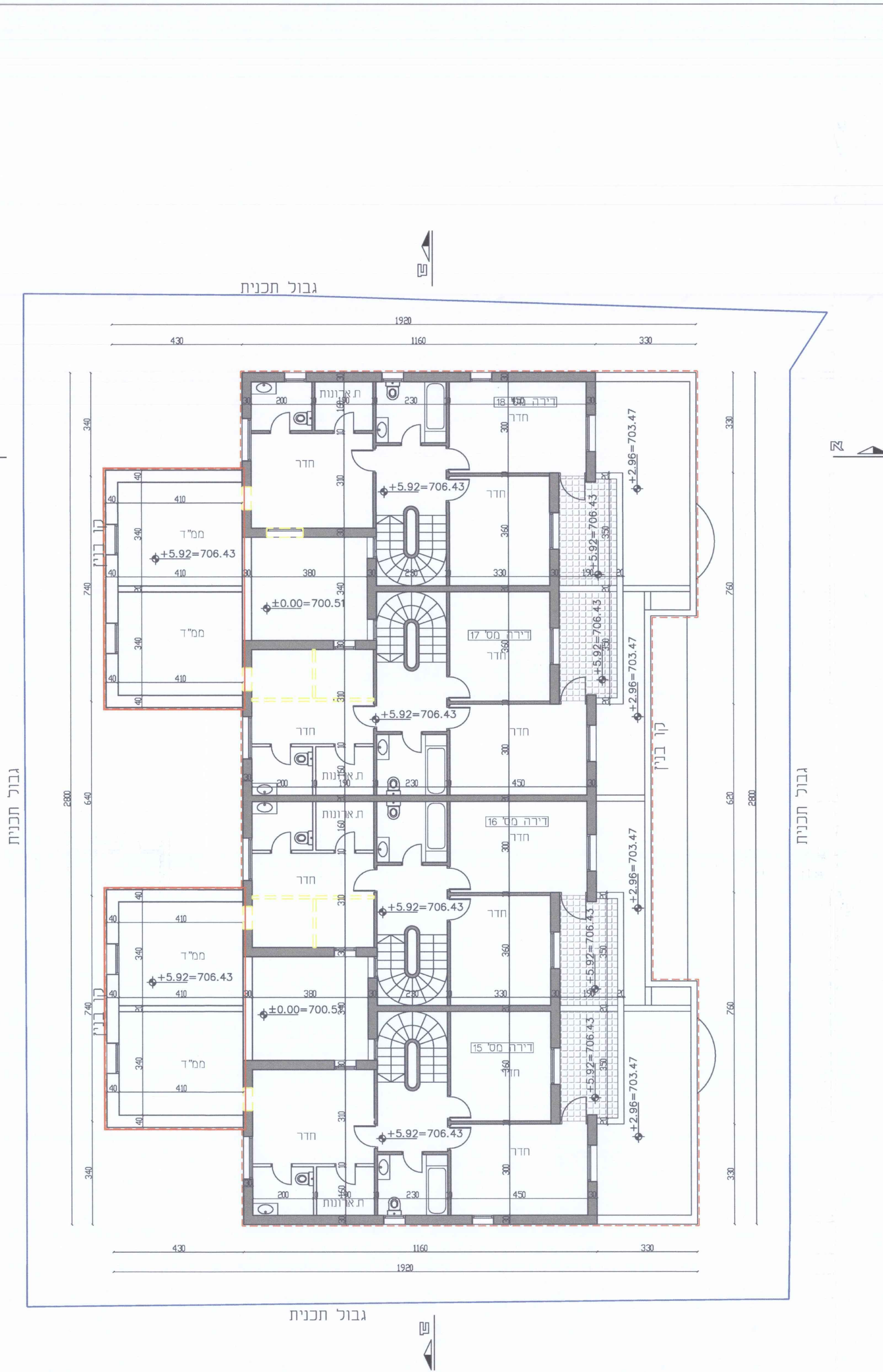
תכנית קומה ב +5.92=706.43 קנ"מ 1:100
