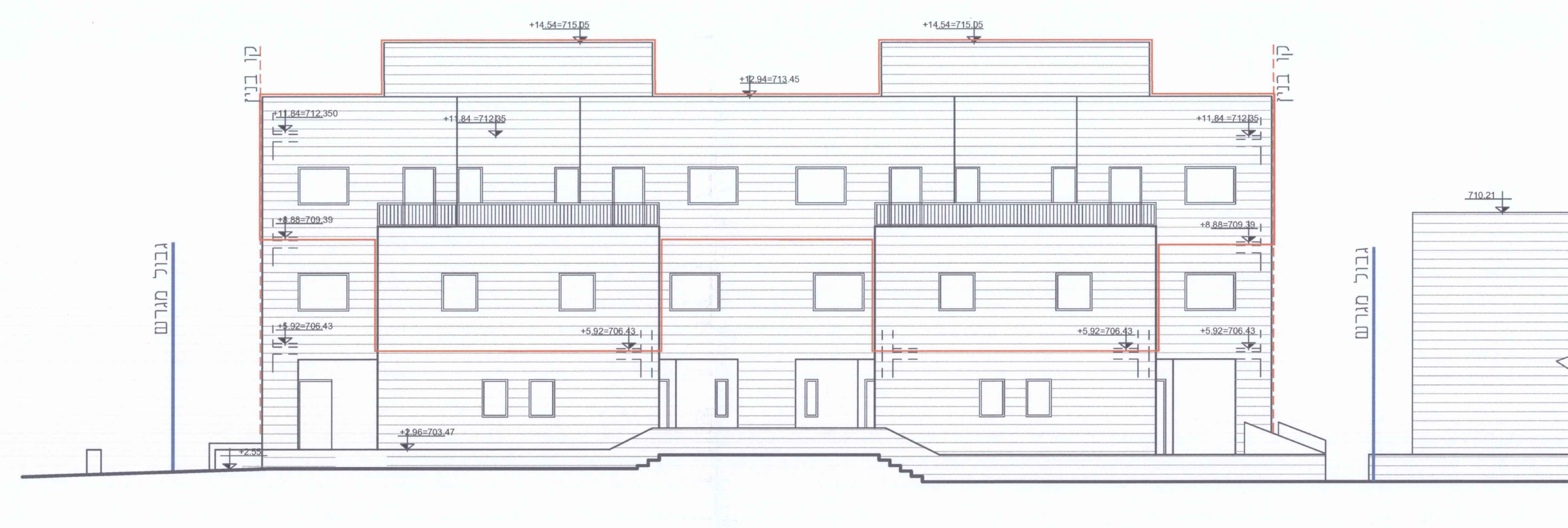
חזית מערבית קנ"מ 1:100
