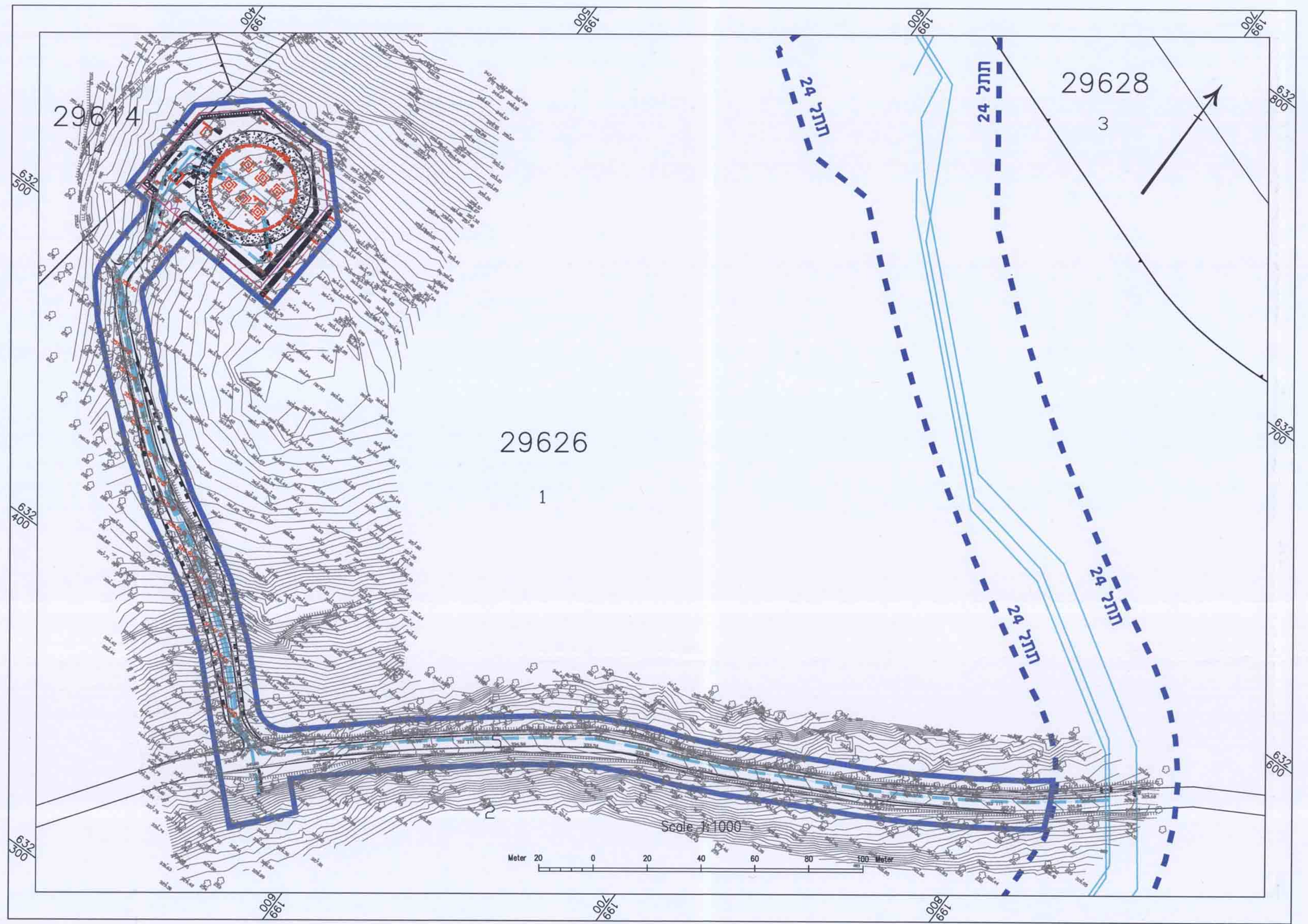
תנוחה כללית קני"מ 1:1,000
