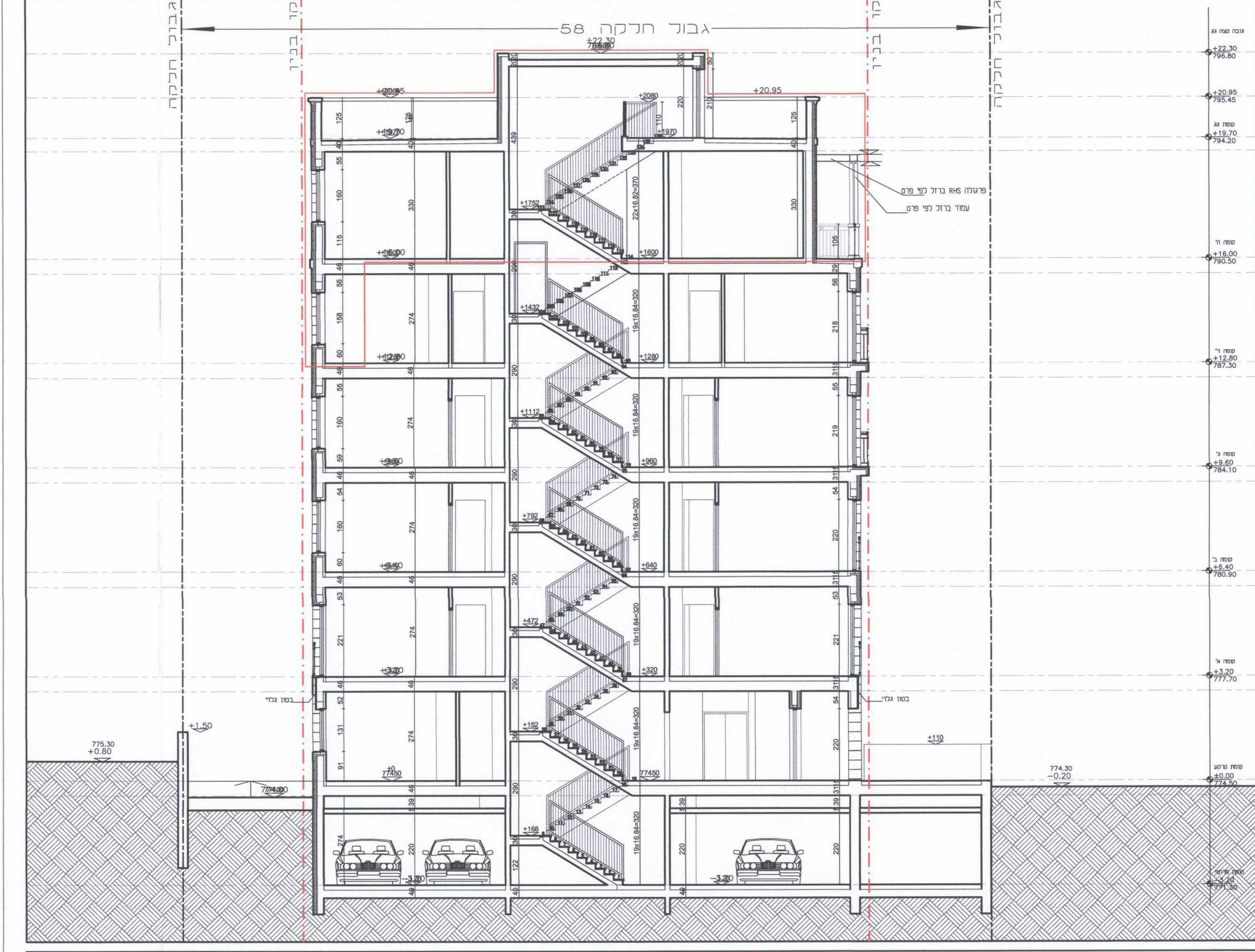
חזית דרומית מזרחית קנ"מ : 1:100
