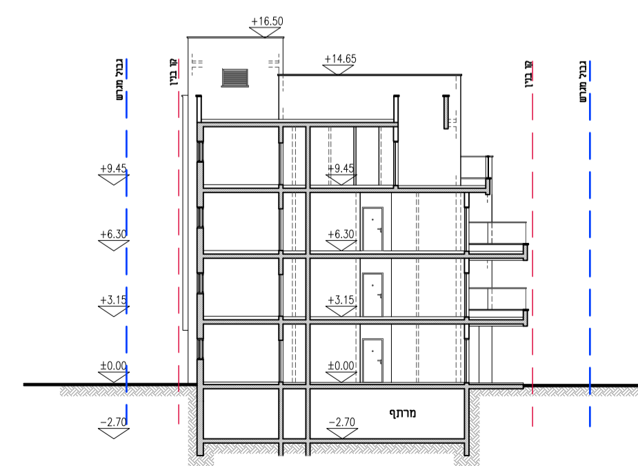
חתך 2-2 קנ"מ 1:250
