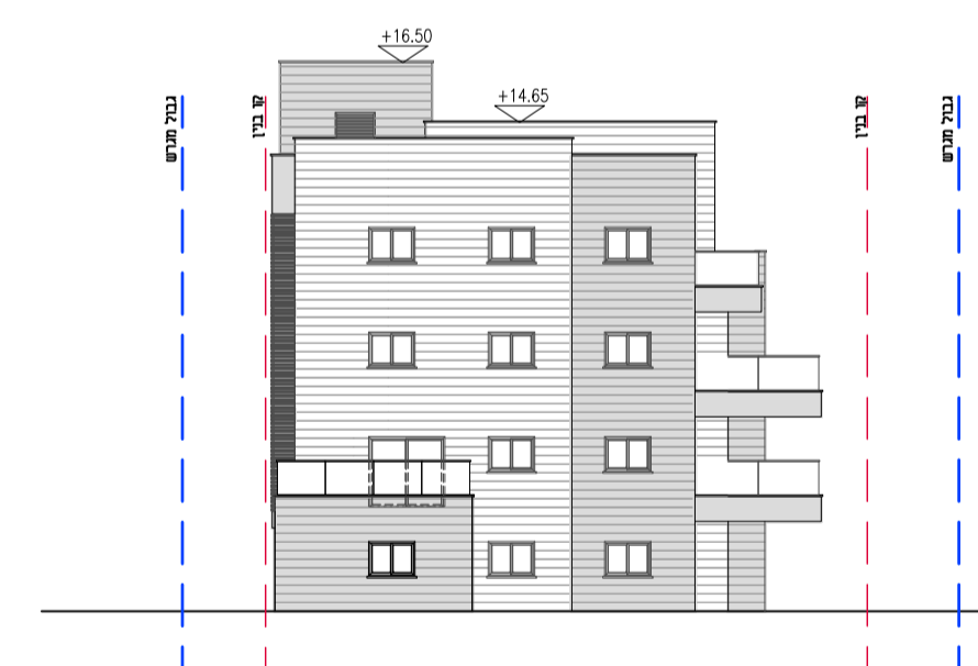
חזית מערבית קנ"מ 1:250
