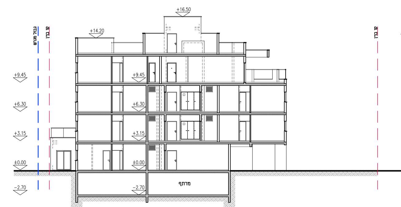
חתך 1-1 קנ"מ 1:250
