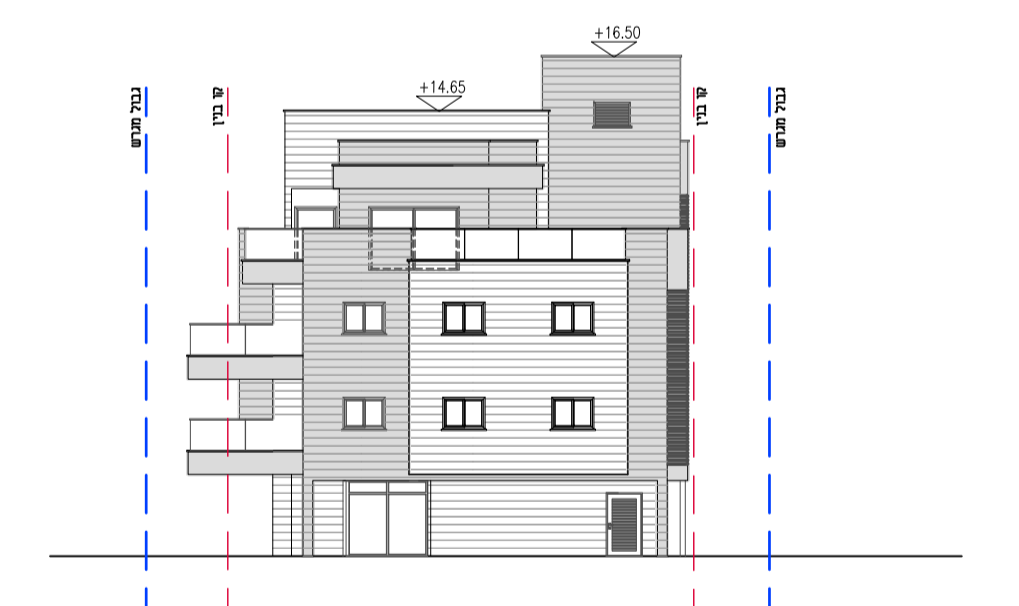
חזית מזרחית קנ"מ 1:250
