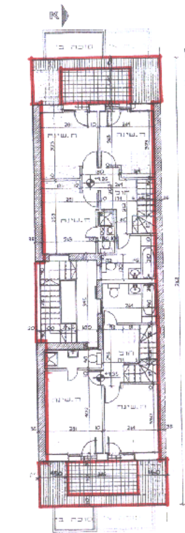
תוכנית קומה ב 1:100
