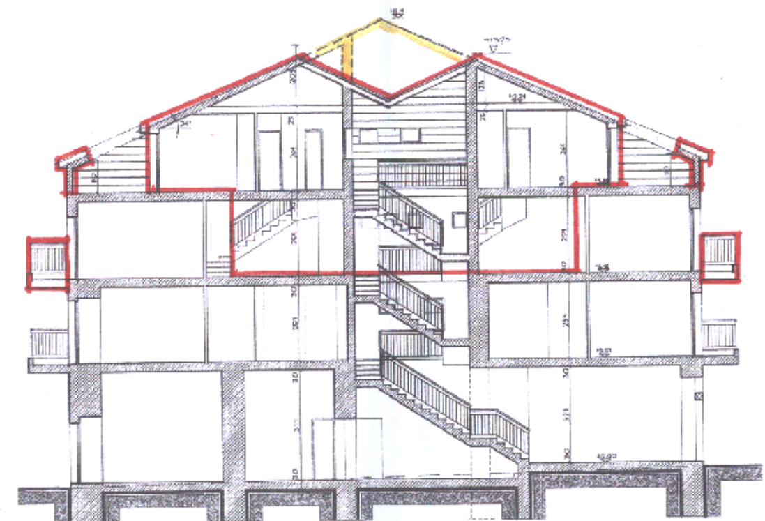
חתך א-א 1:100
