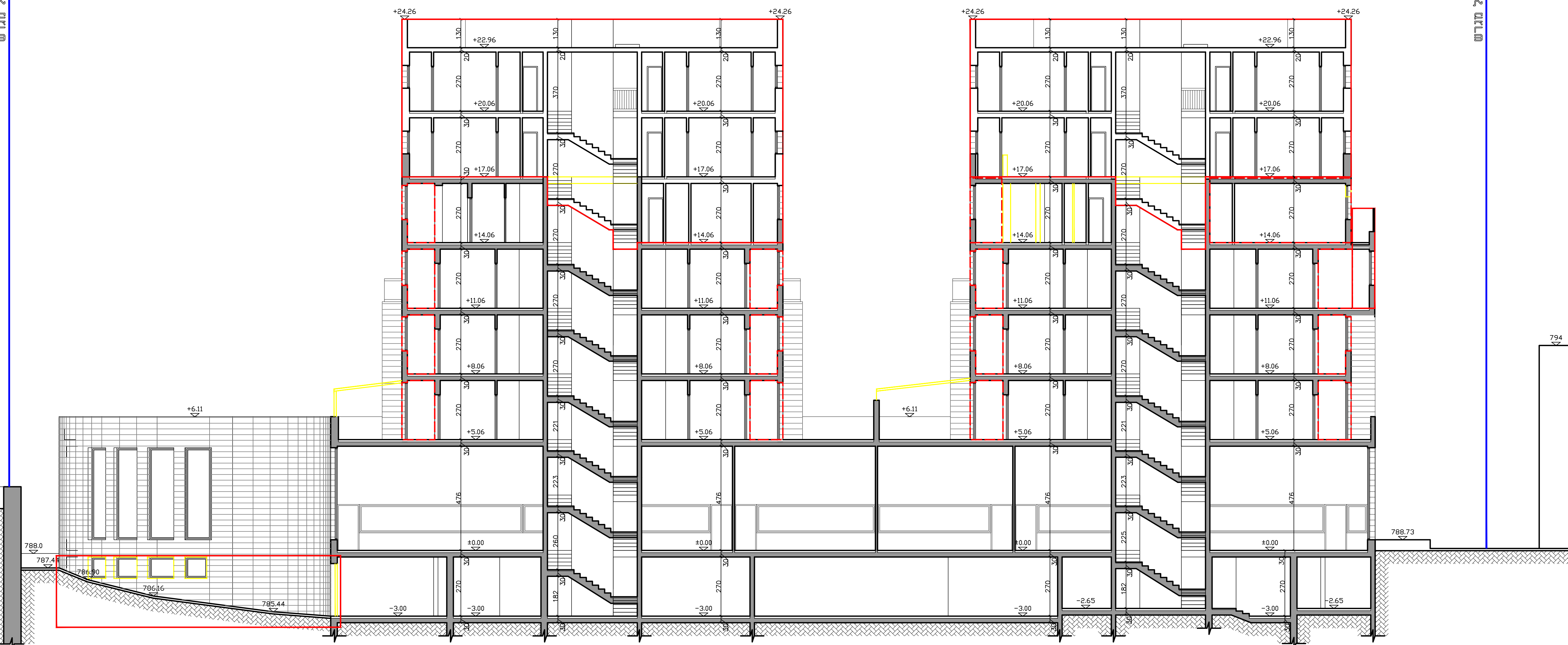
חיתך ב-ב קני"מ 1:100
