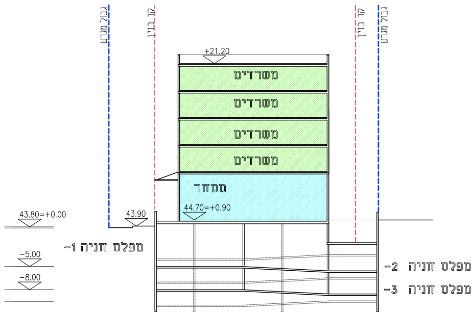
חתך עקרוני 2-2 קני"מ 1:500
