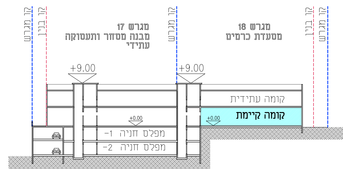
חתך 1-1 קנ"מ 1:500
