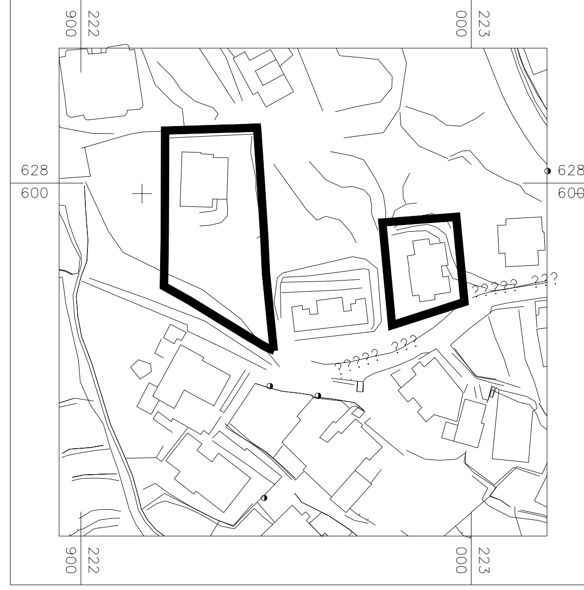
תרשים המקום ק"מ 1:1250
