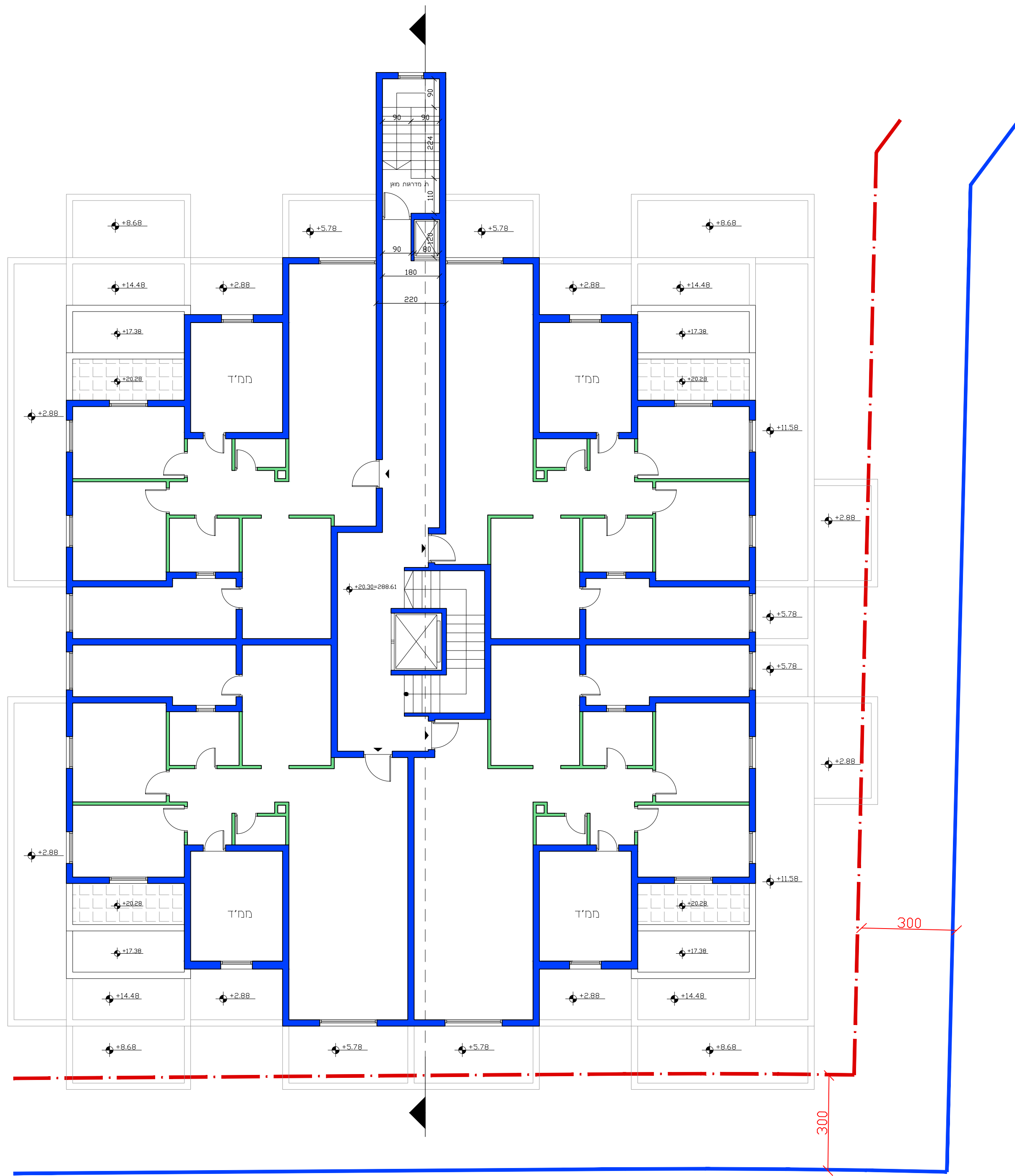
תכנית קומה ז'
