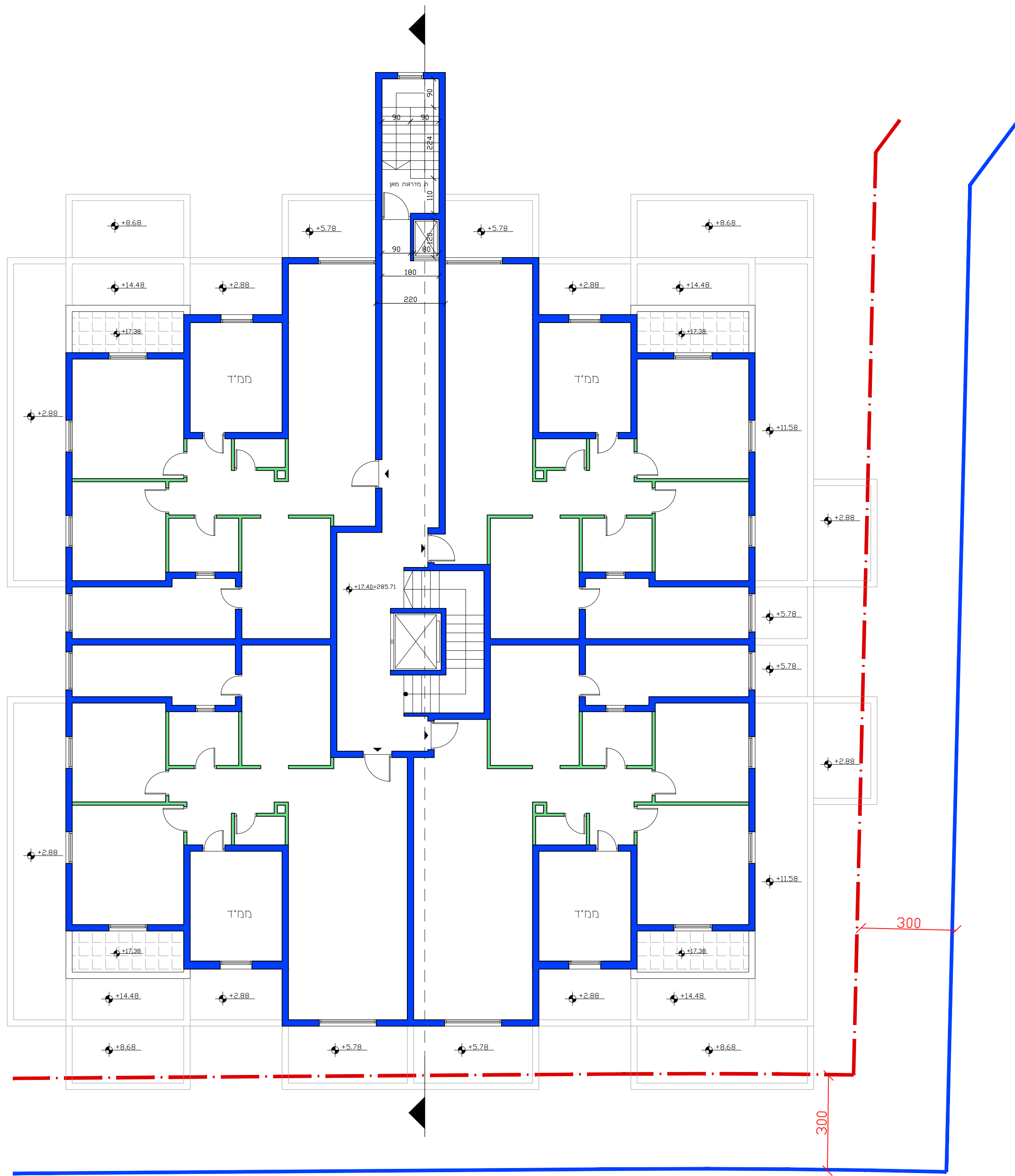
תכנית קומה ו'
