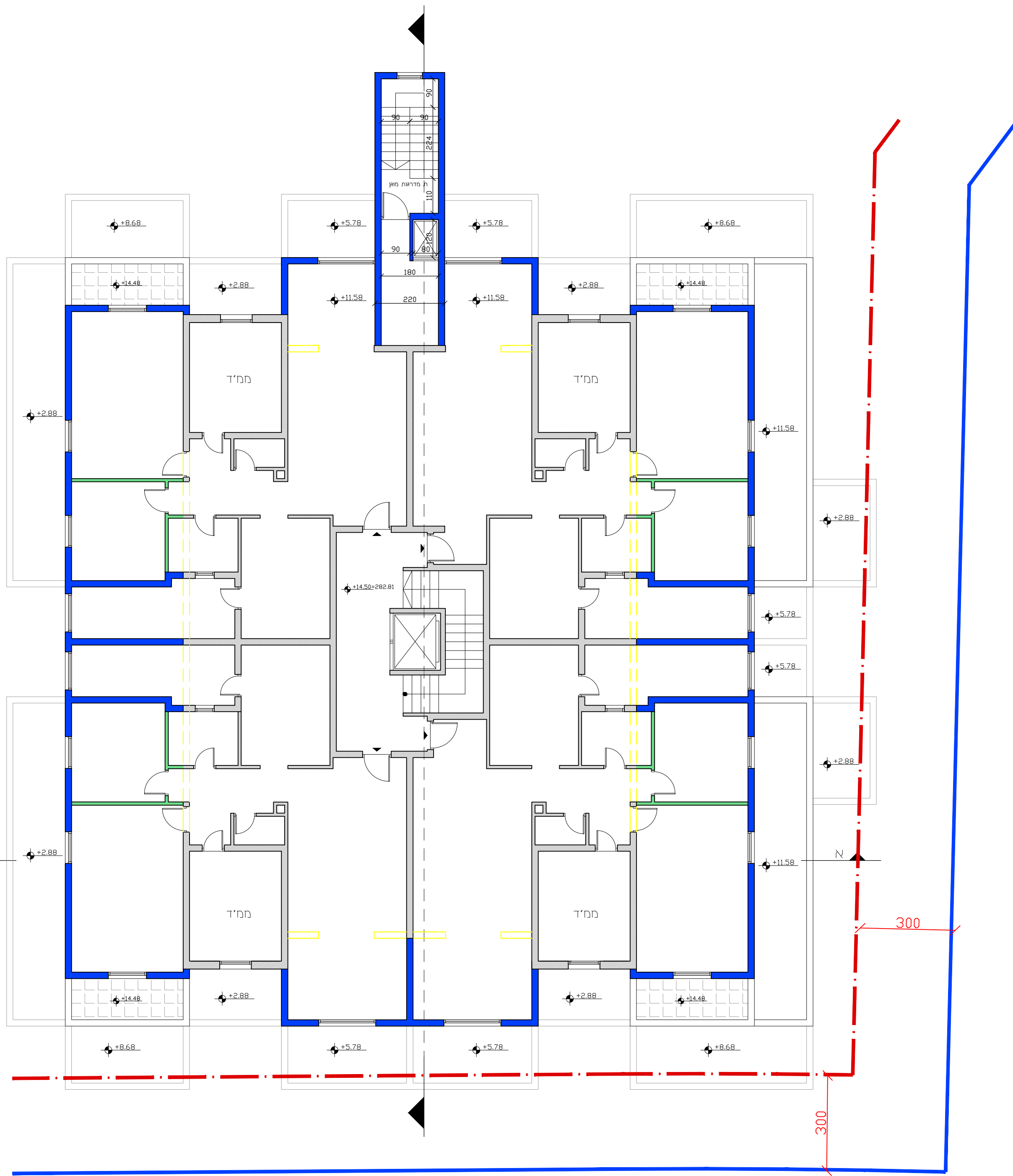
תכנית קומה ה'
