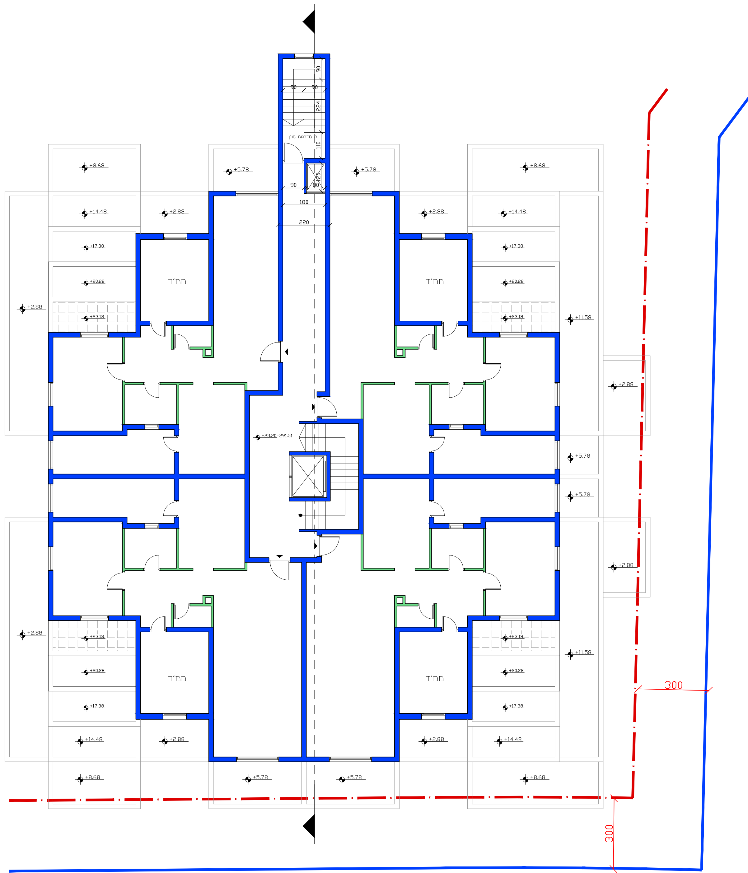
תכנית קומה ח'
