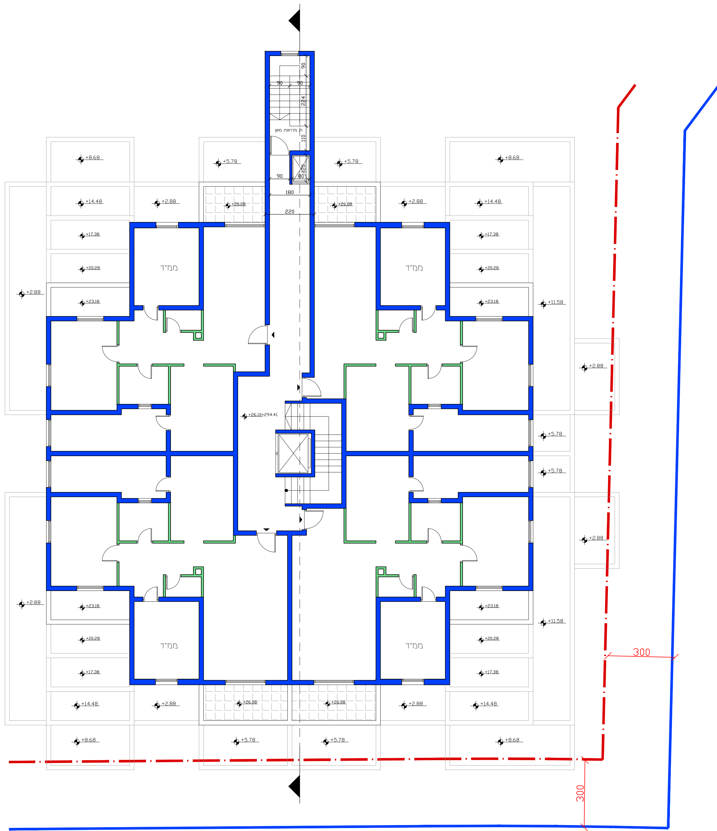
תכנית קומה ט'
