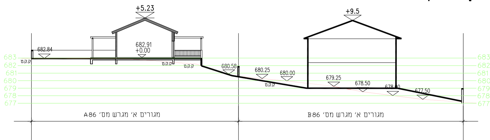
חתך 1-1 קני"מ 1:250
