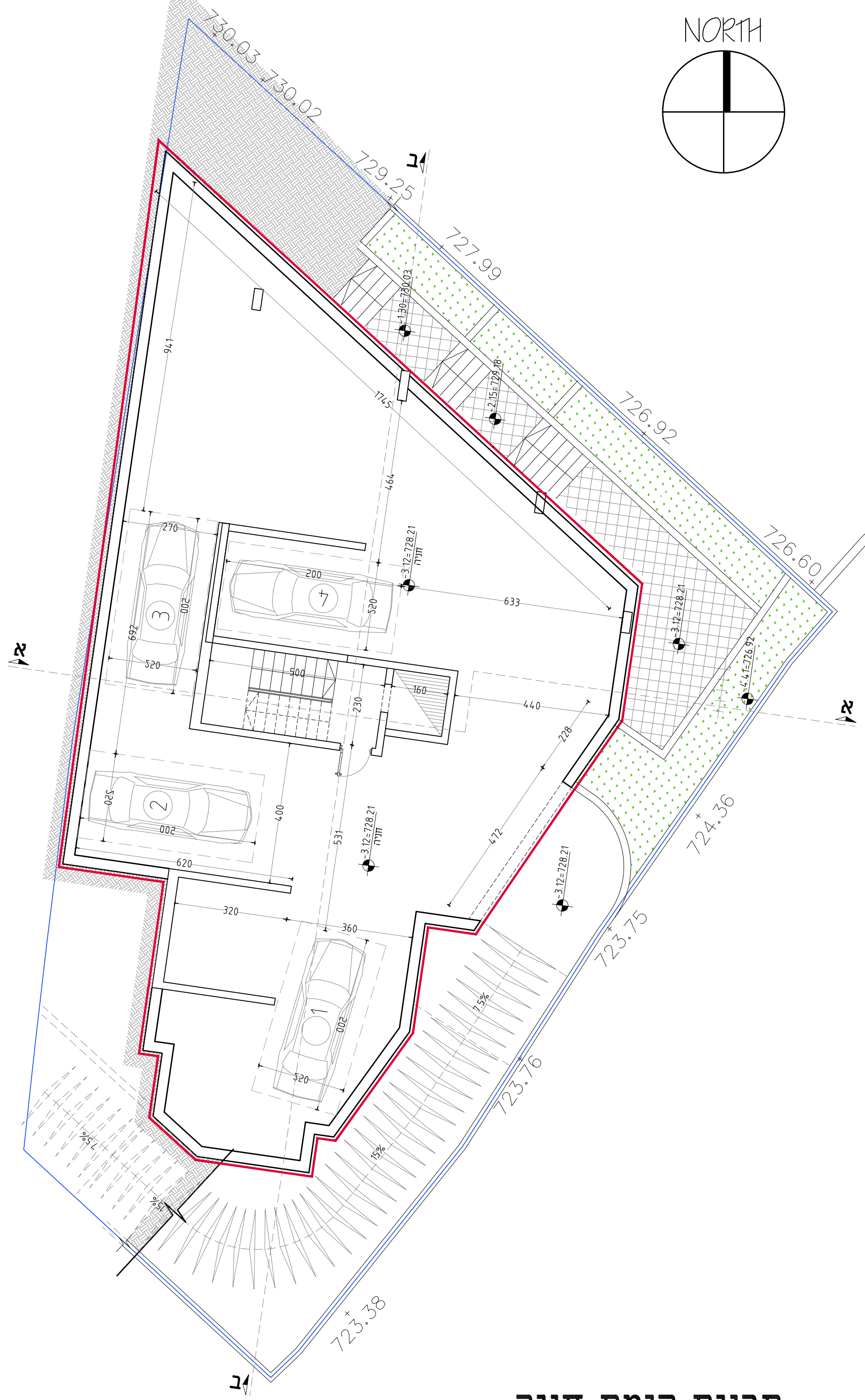
תכנית קומת חניה ק.מ. 1:100
