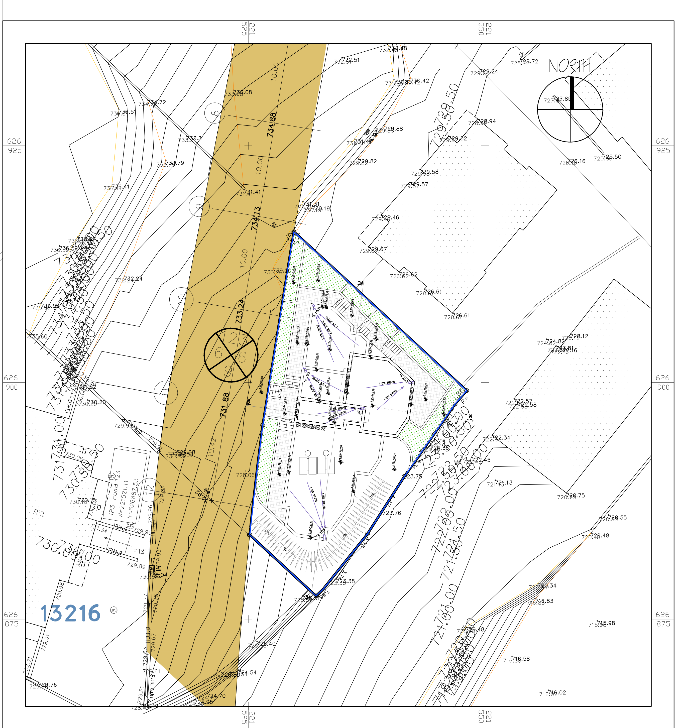
תכנית פיתוח השטח ק.מ. 1:200
