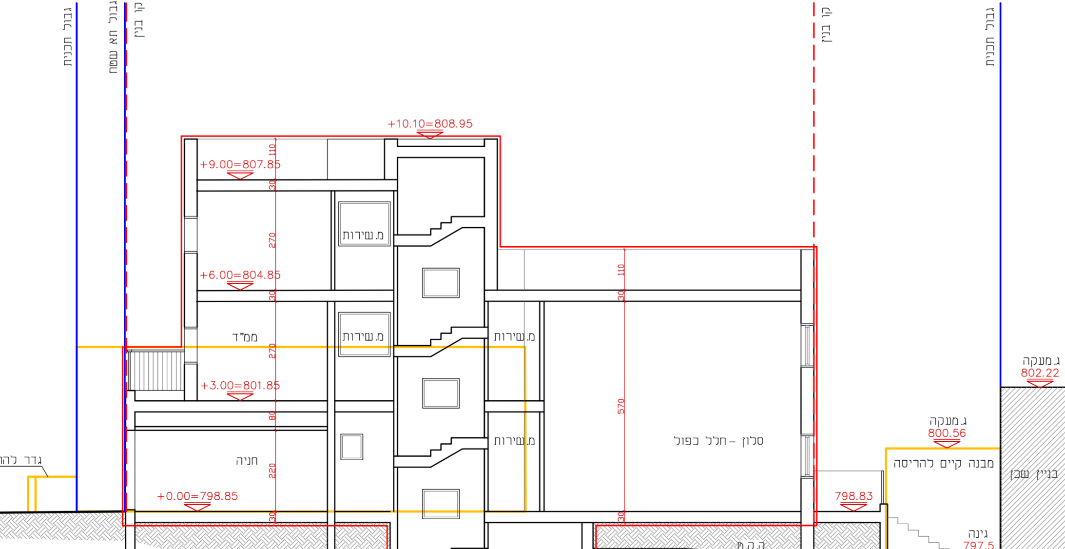
חתך א - א ק.מ. 1:100
