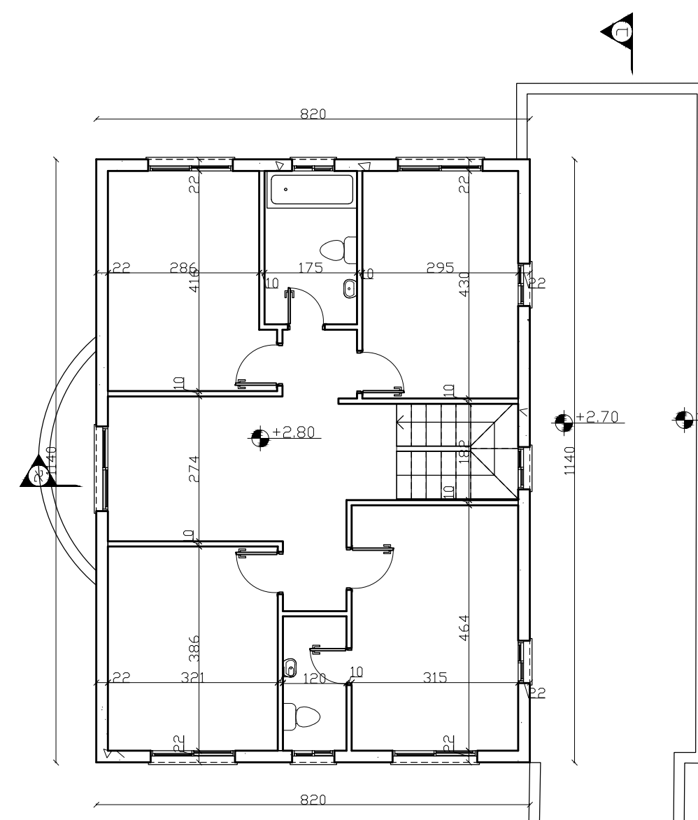
תכנית קומת קומה א' מפרס +2.80 (+262.39) קנ"מ 1:100
