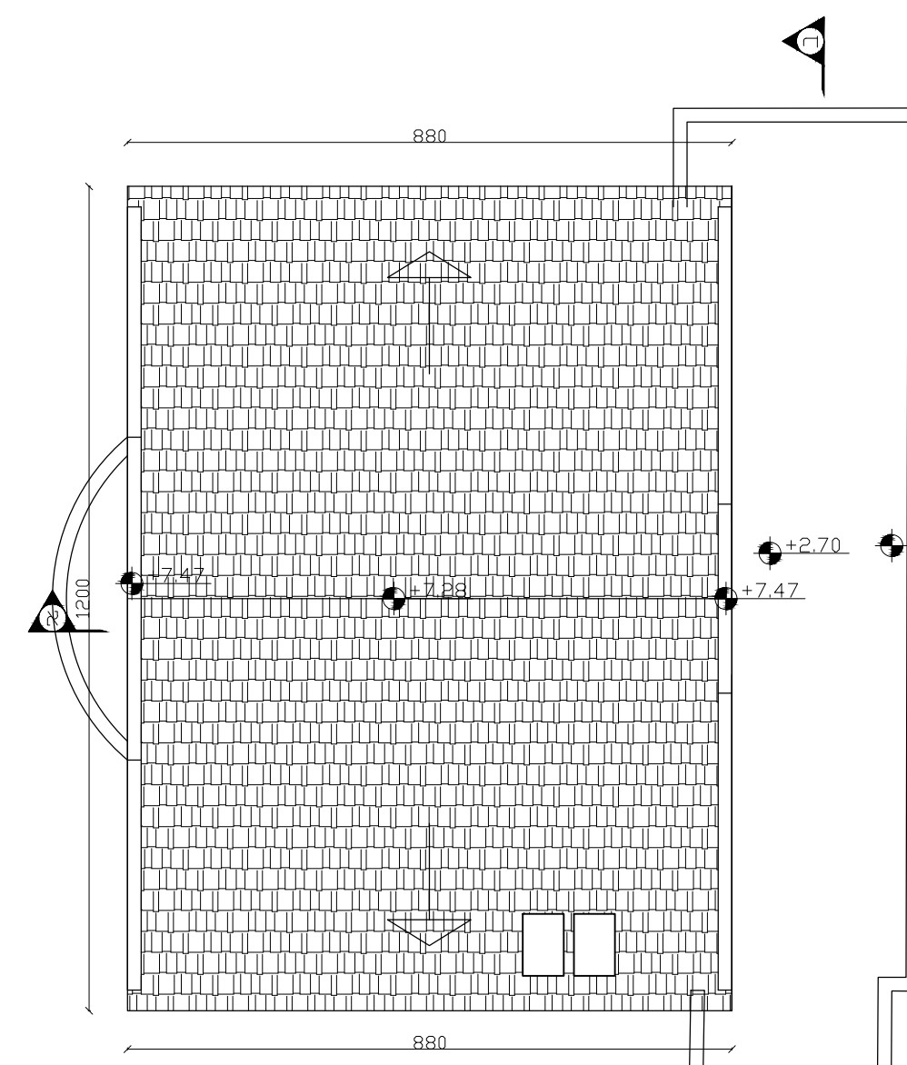
תכנית גגות מפרס +7.28 (+266.81) קנ"מ 1:100
