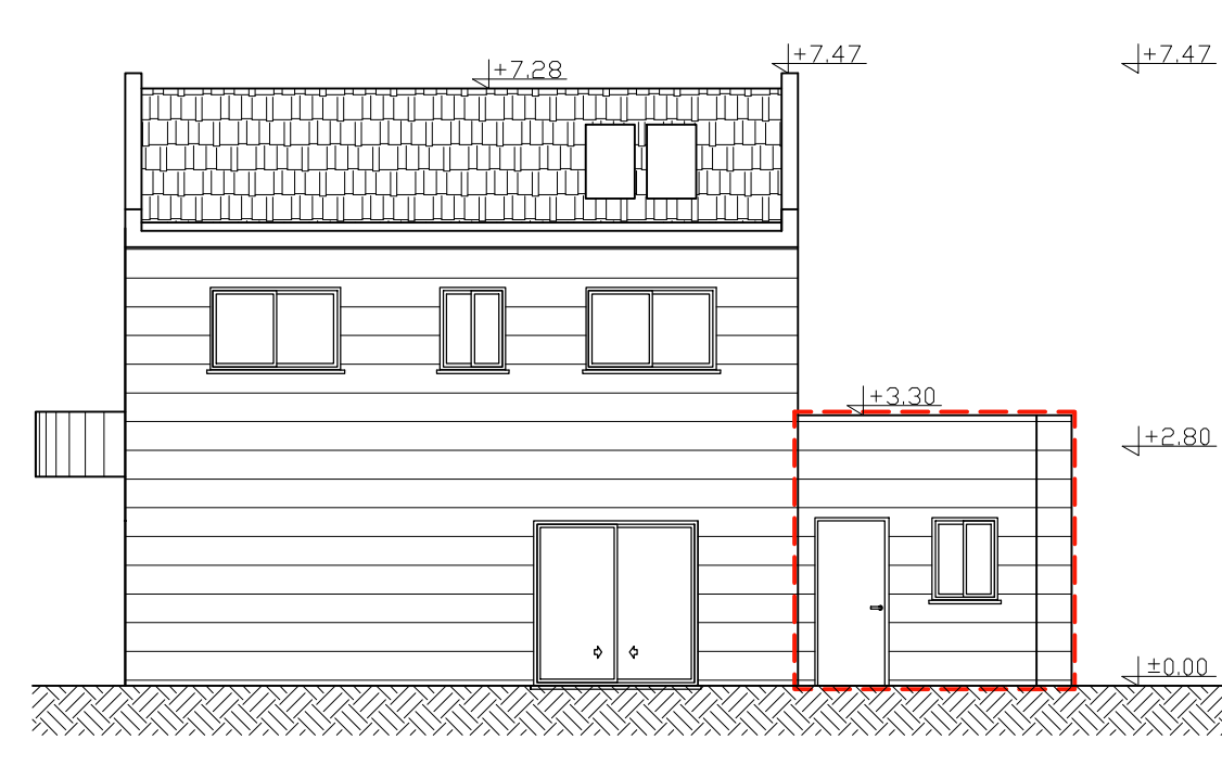
חזית דרומית קנ"מ 1:100
