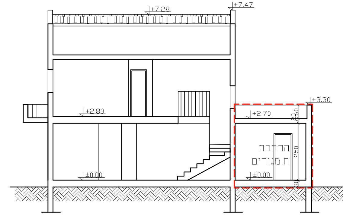
חתר א' א' קנ"מ 1:100
