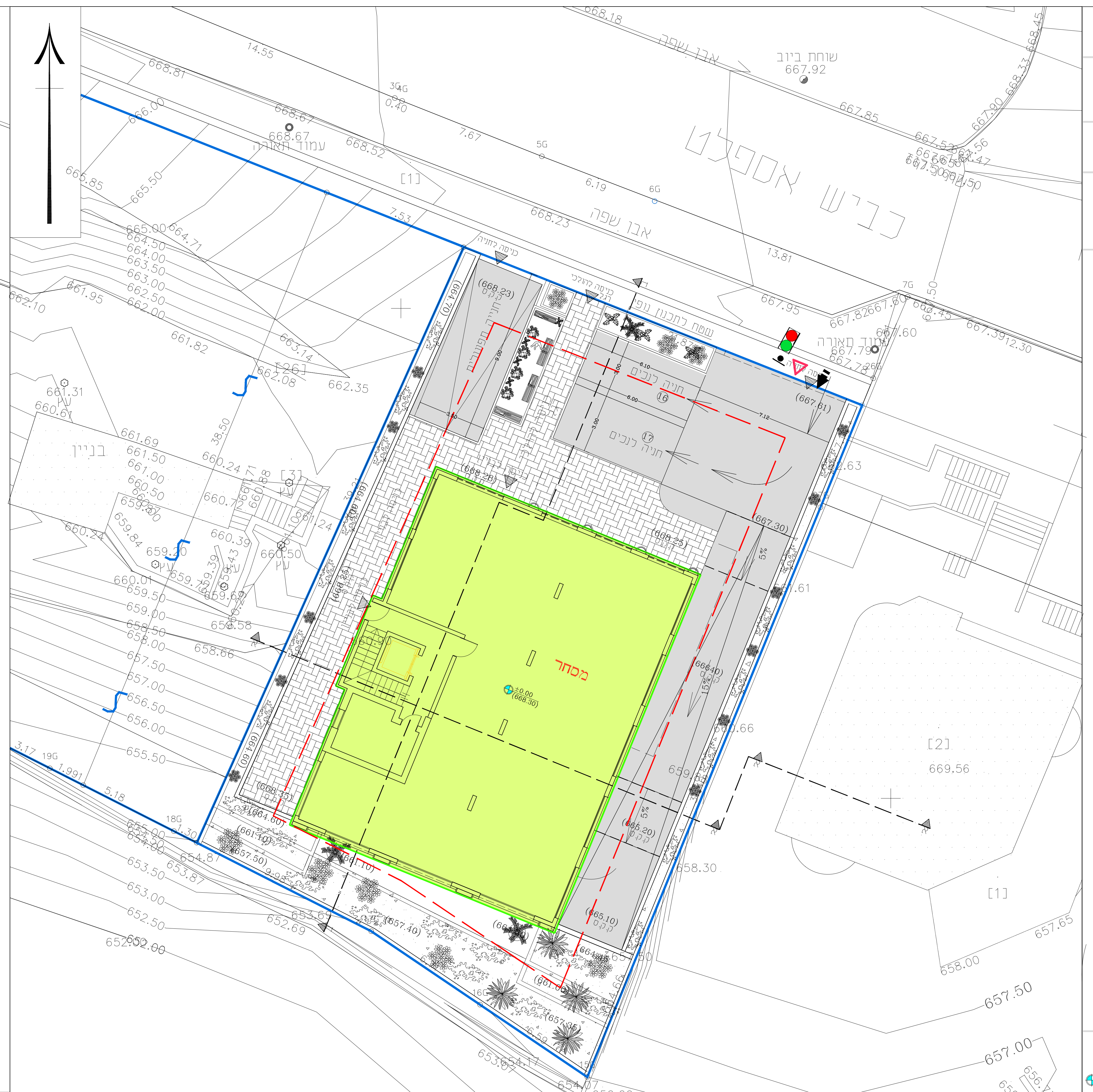
תכנית פיתוח קנ"מ 1:100 מפלס \pm 0.00 (668.30) תכנית קומת קרקע קנ"מ 1:100 מפלס \pm 0.00 (668.30)
