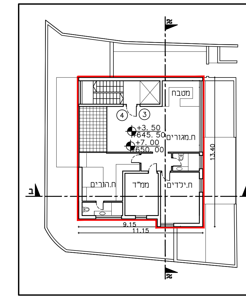
תכנית קומה א', ב'
