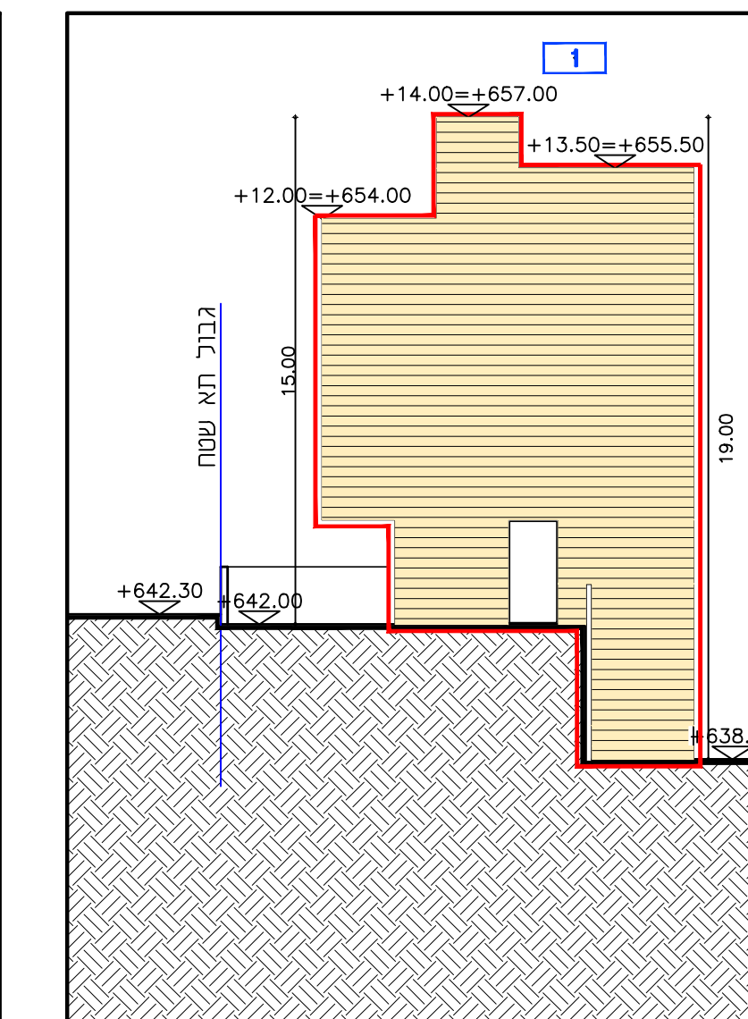
חזית צפונית
