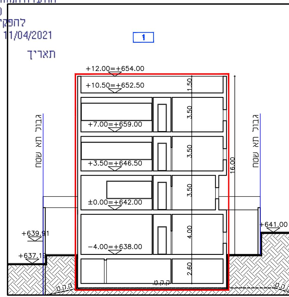
חתך א-א
