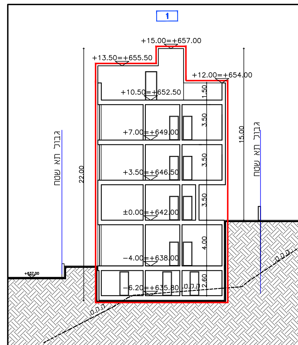
חתך ב-ב
