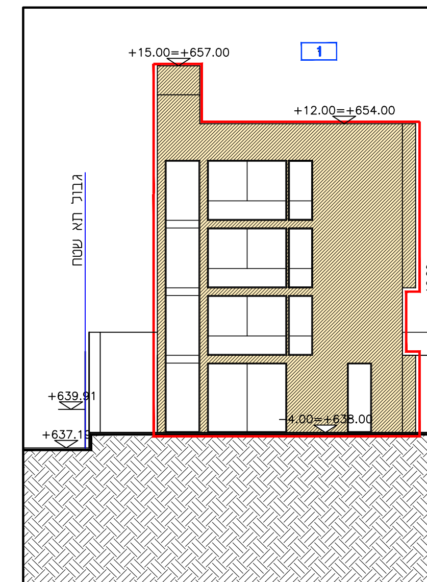
חזית מערבית
