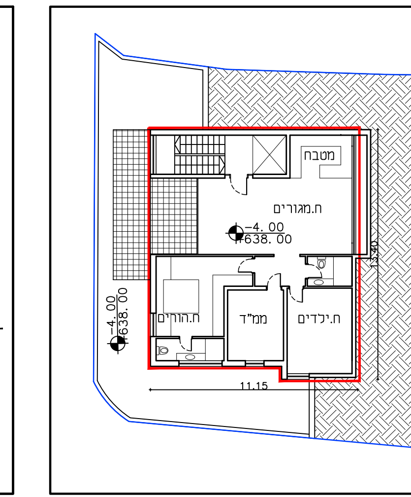
תכנית קומת -1
