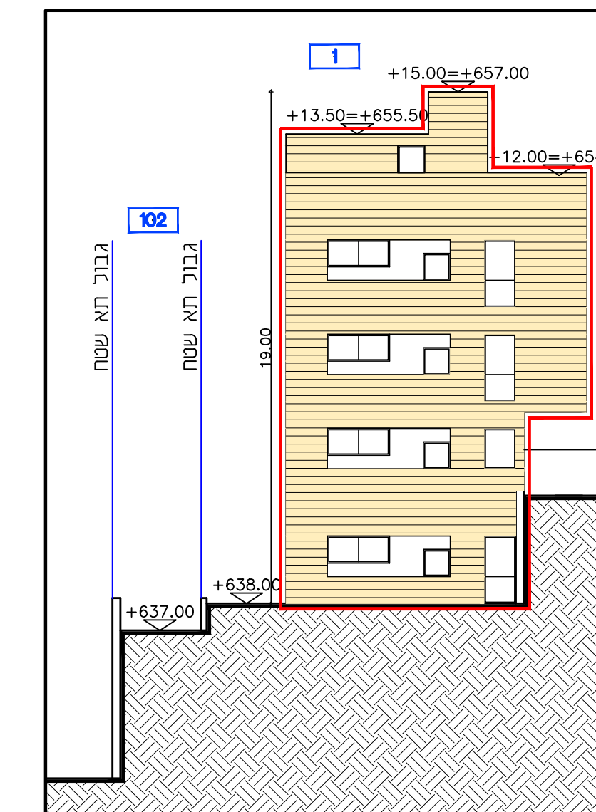
חזית דרוםית
