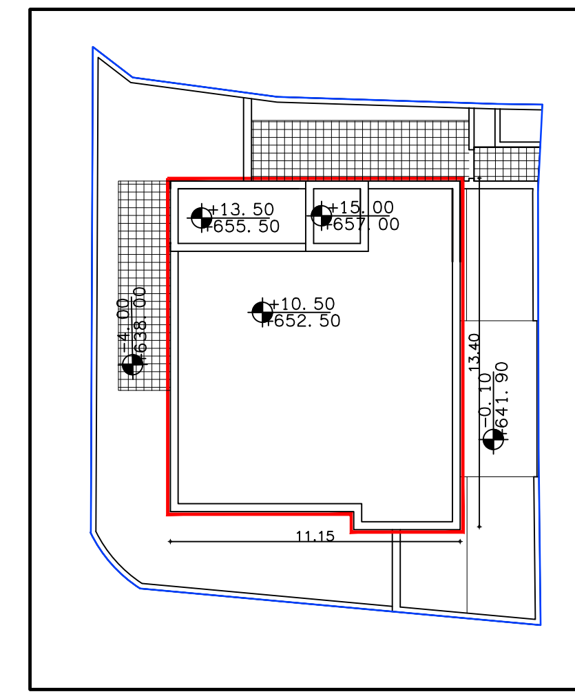
תכנית קומת גג
