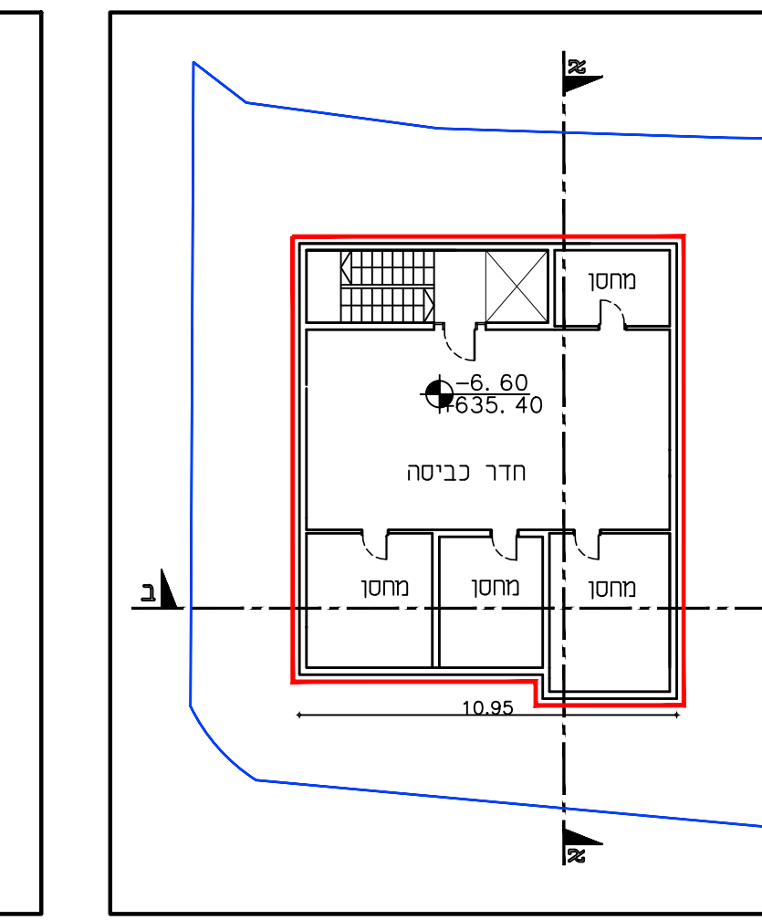
תכנית קומת -2
