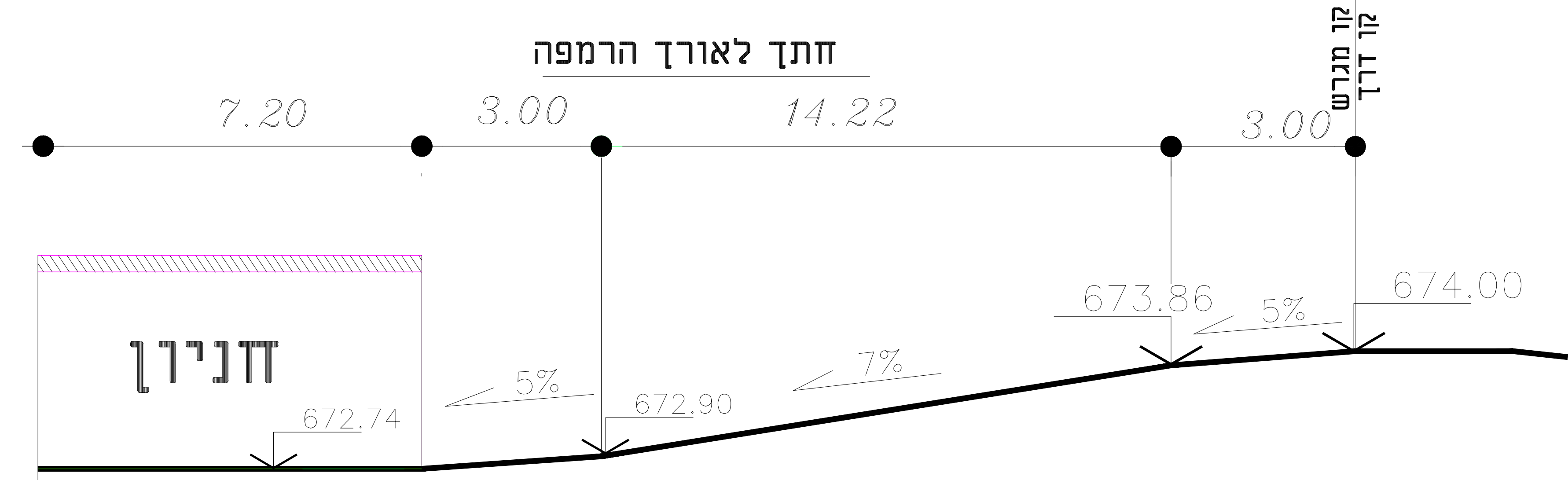
תכנית קומת חניה תת קרקעית קנ"מ 1:100 מפלס (-2.53 / 672.74)
