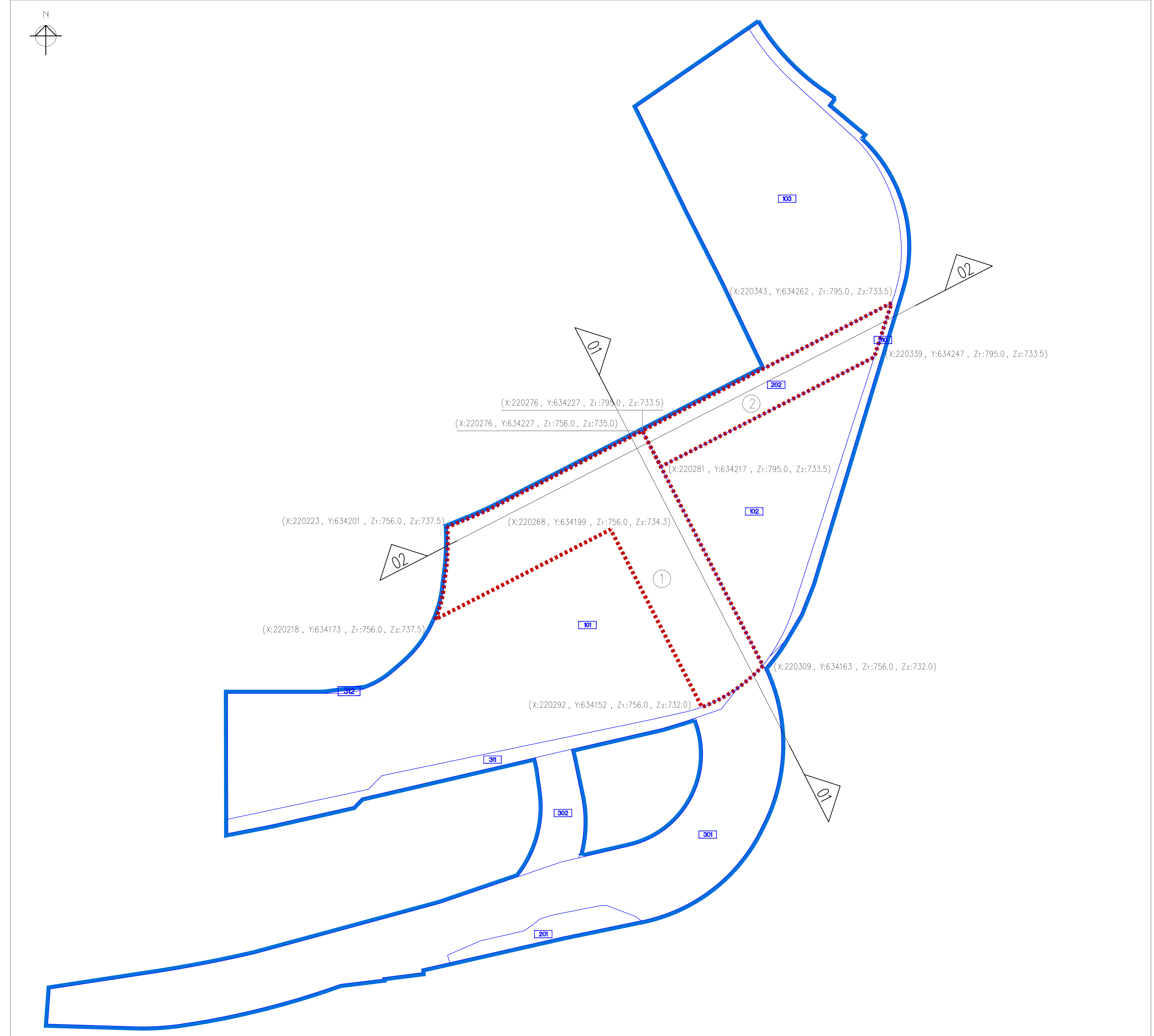
תשריט מצב מוצע
