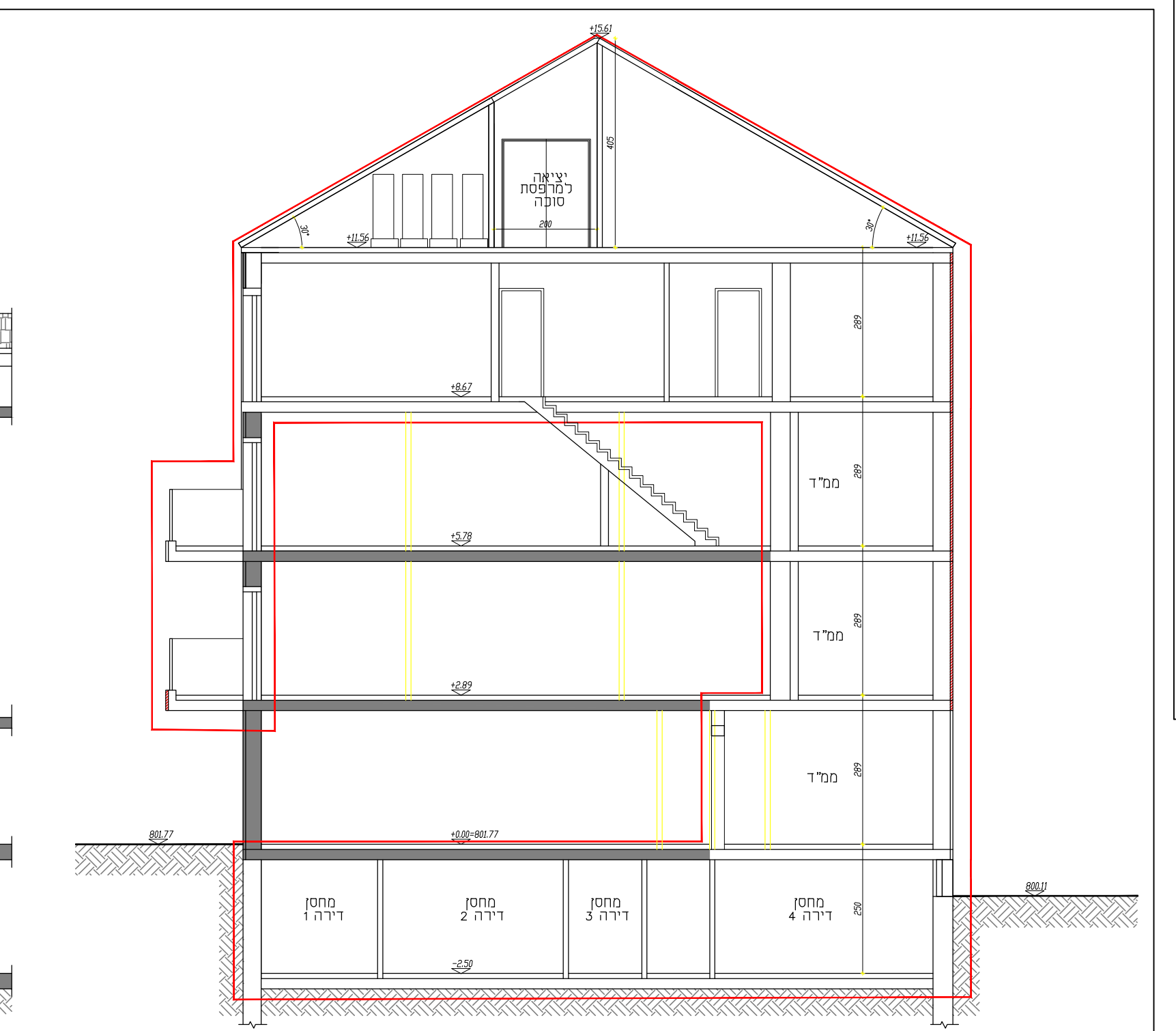
חתך א-א קנ"מ: 1:100
