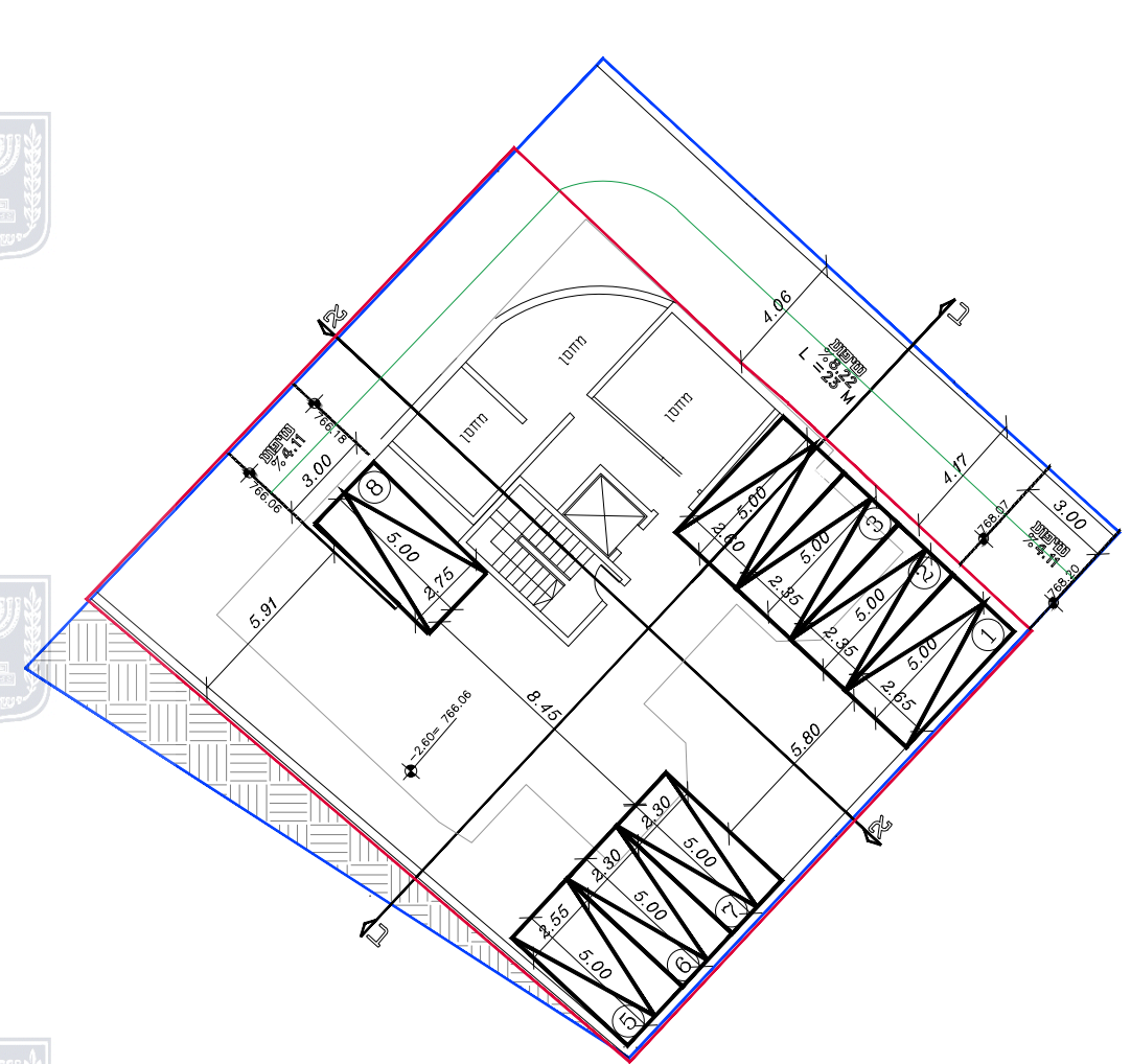
תכנית קומת מרתף מ.ס. 1-280
