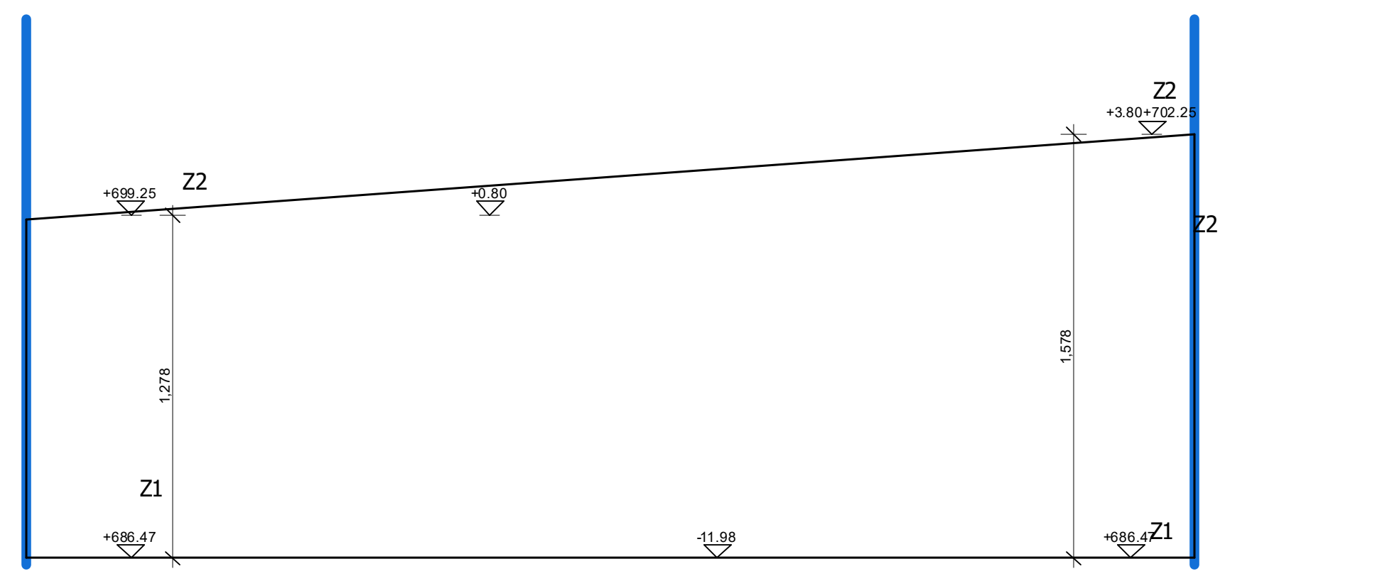
חתך 1-1 1:200
