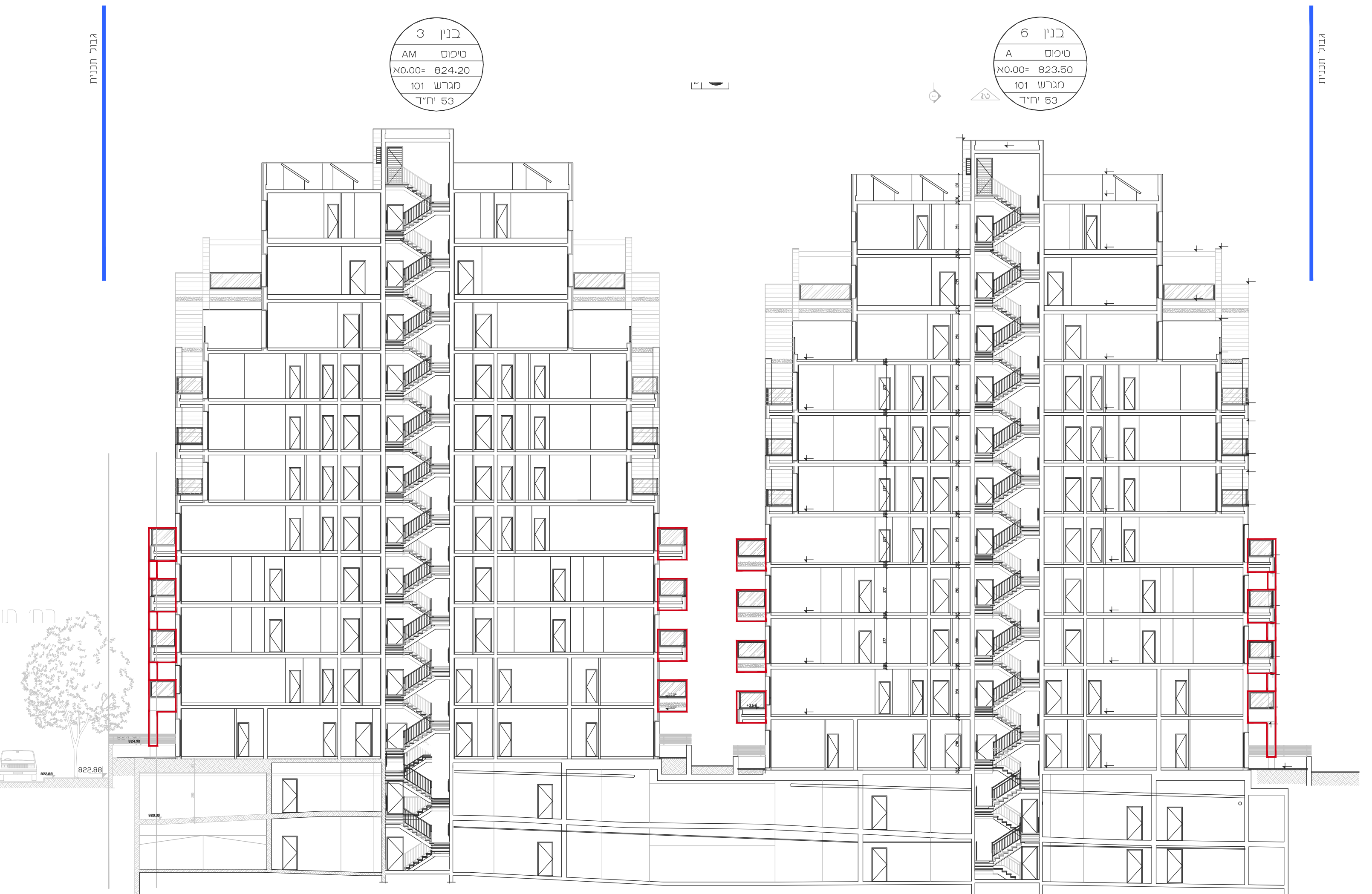
חתך 1-1
