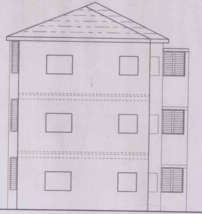
תז'ית דרום'ית ק.מ. 1:100
