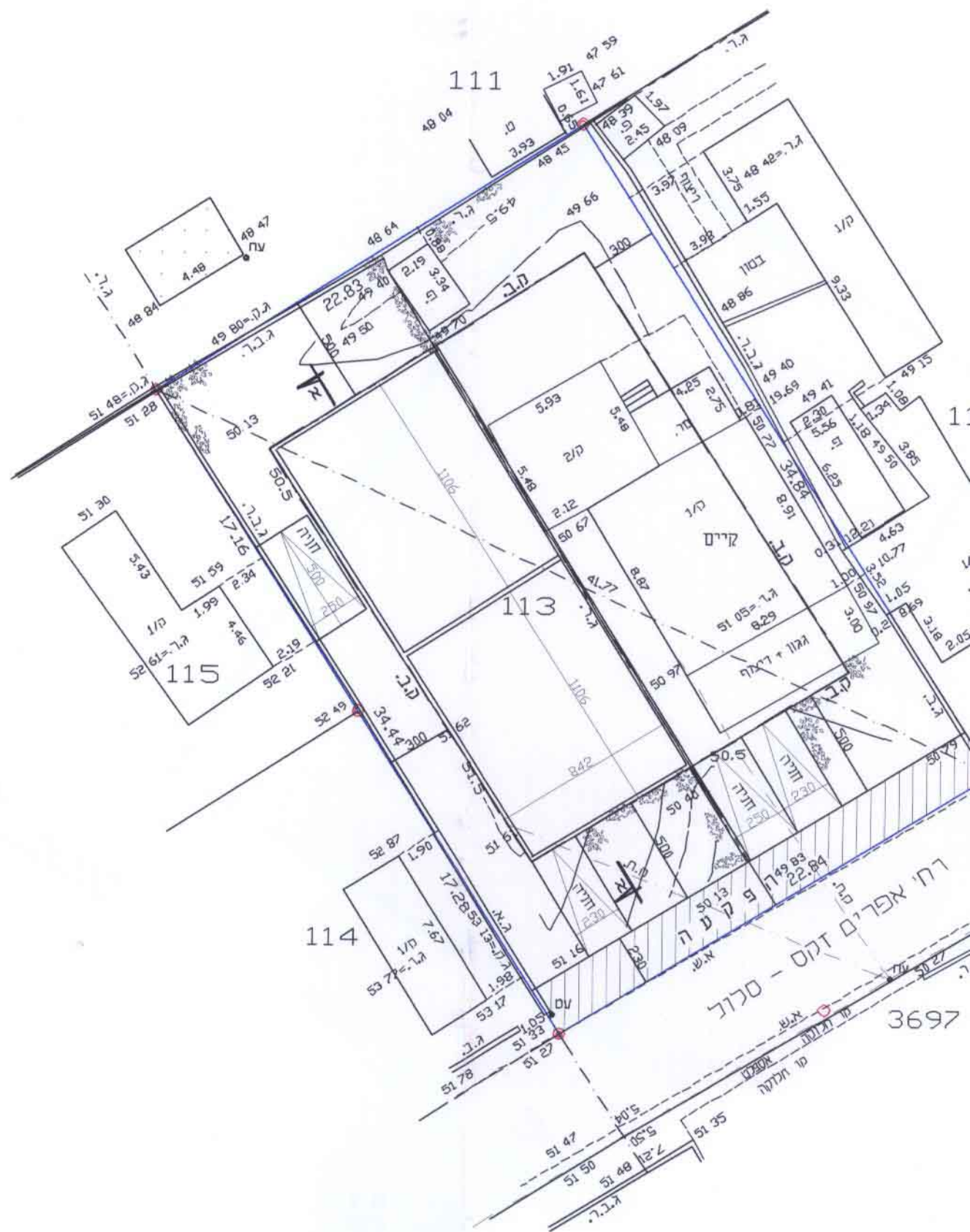
בינוי סכמטי ק. קרקע ק.מ. 1 : 250
