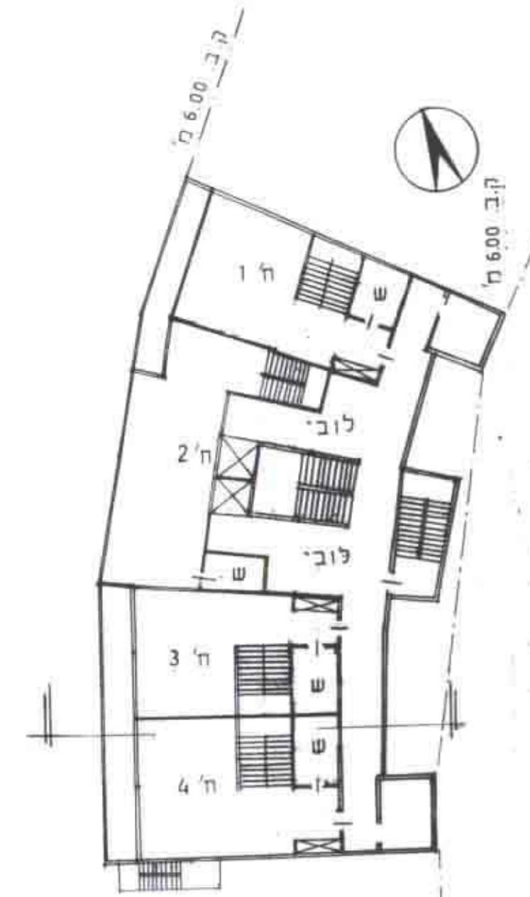
תכנית קומה ח' מפלס תחתון ק.מ. 1/250
