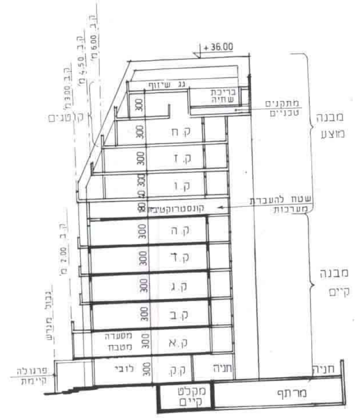
חתך טיפוסי ק.מ. 1/250
