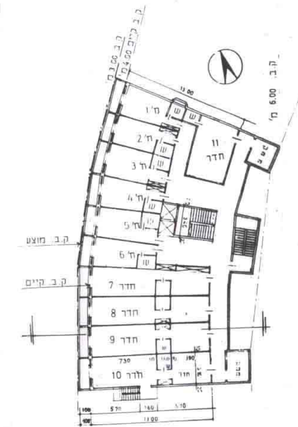
תכנית קומות ב ג ד ה ק.מ. 1/250 (שיפוף קומות קיימות)
