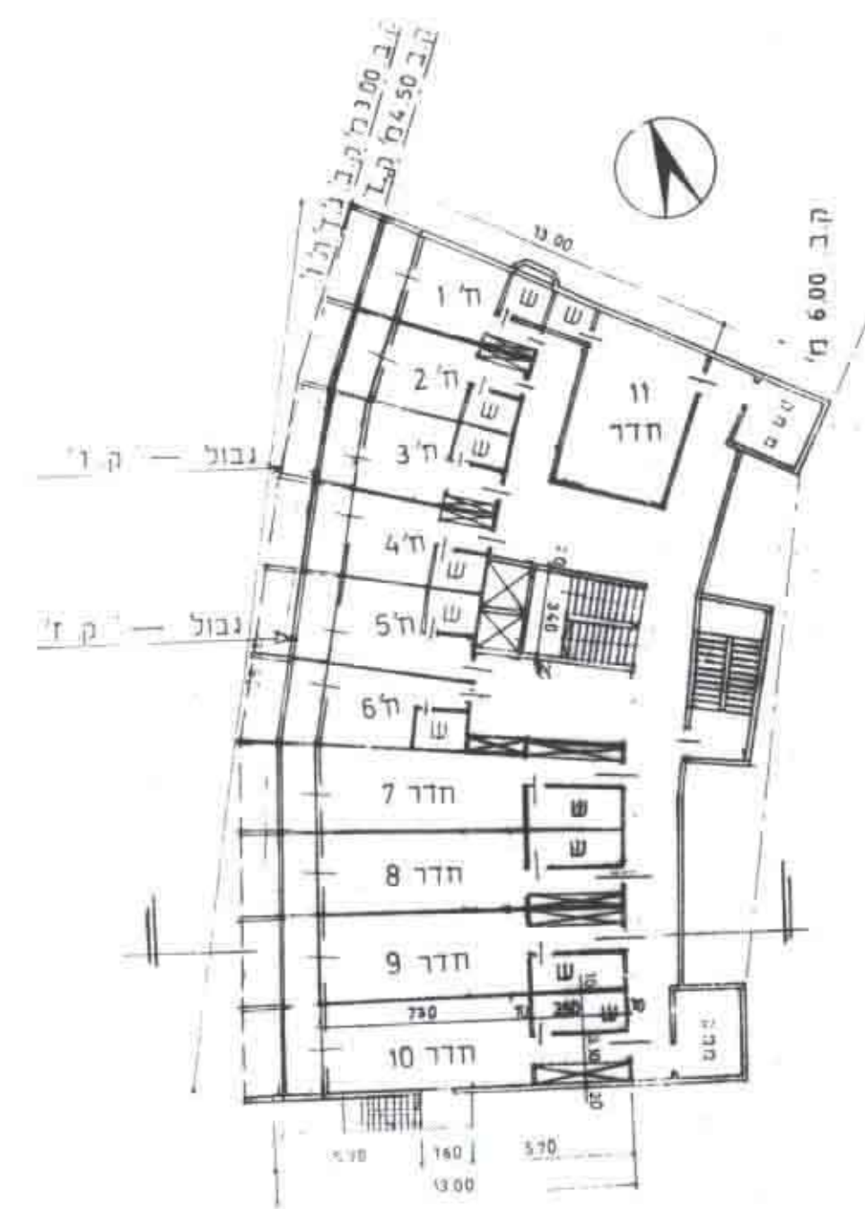
תכנית קומות ו ז' מוצעות ק.מ. 1/250
