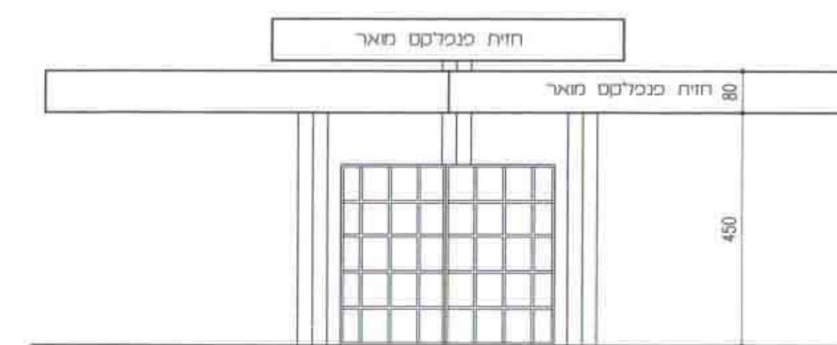
חזית דרומית
