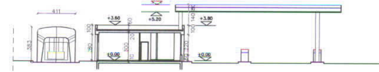
חתך 1-1 ק.מ. 1:250
