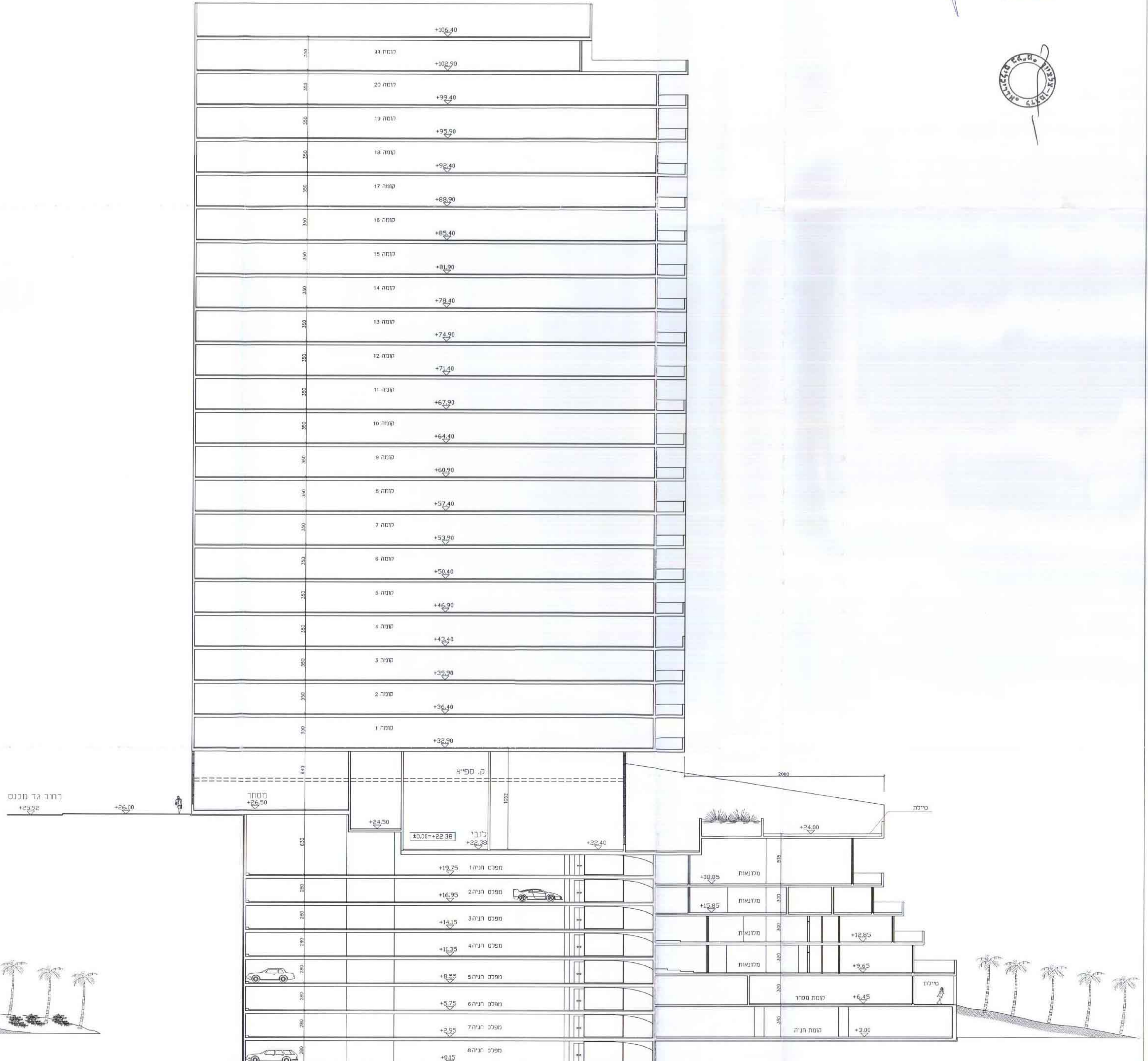
חתך א-א ק.מ. 1:200
