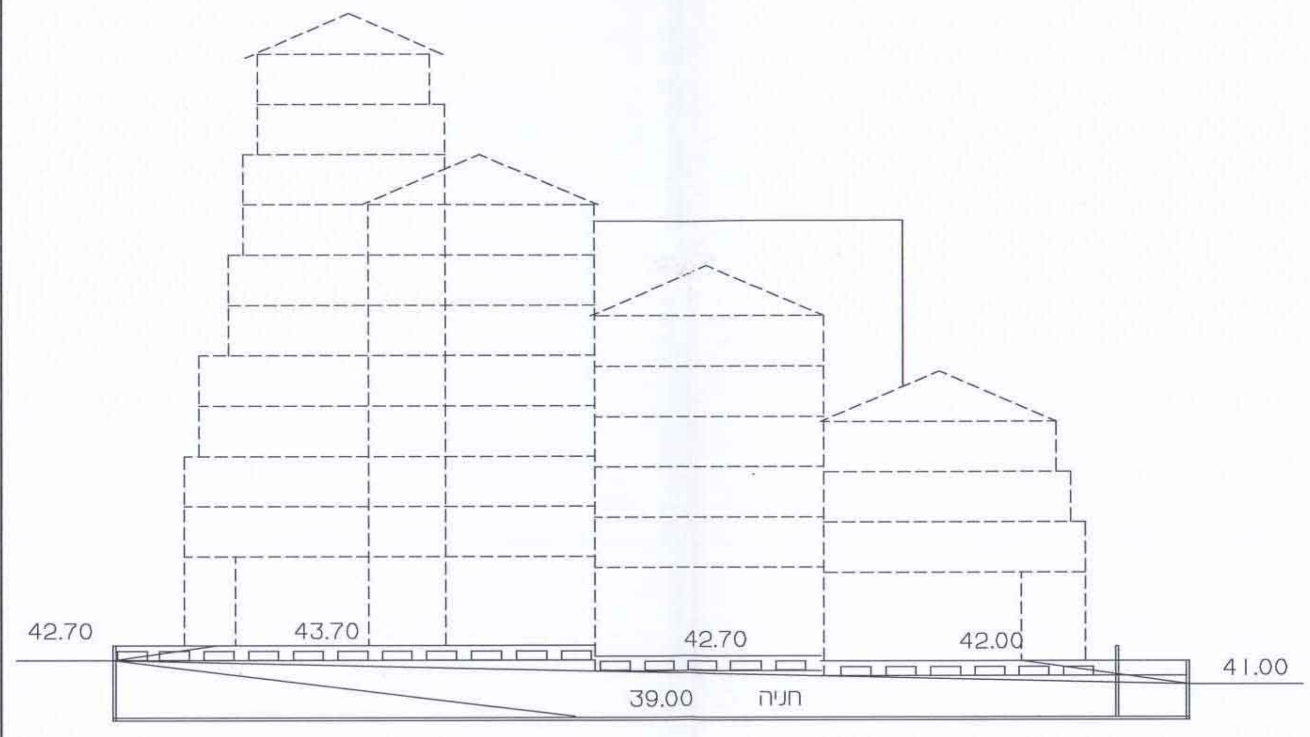
חתך F-F
