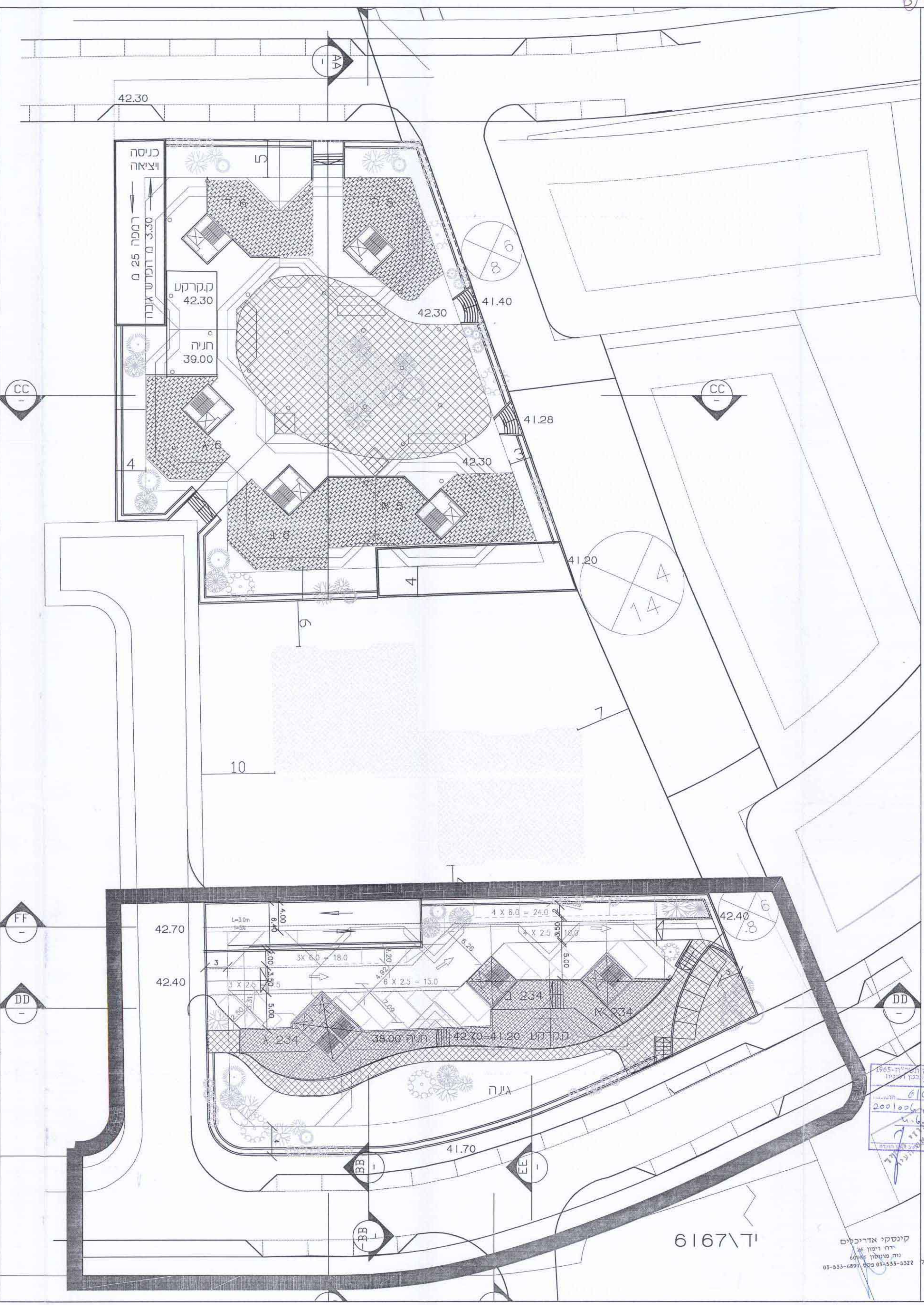
1) תכנית מפלס הקרקע
