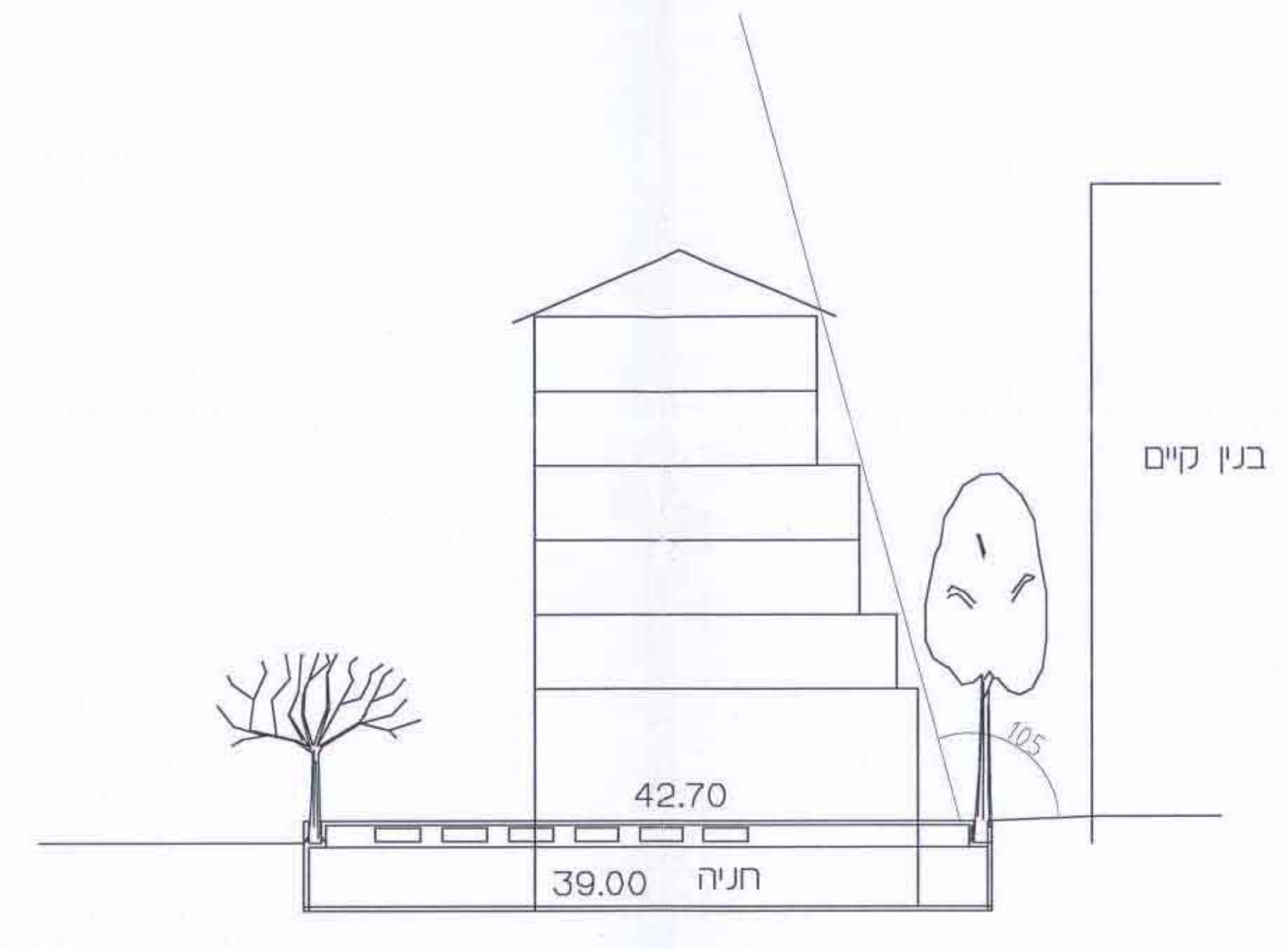
חתך E-E
