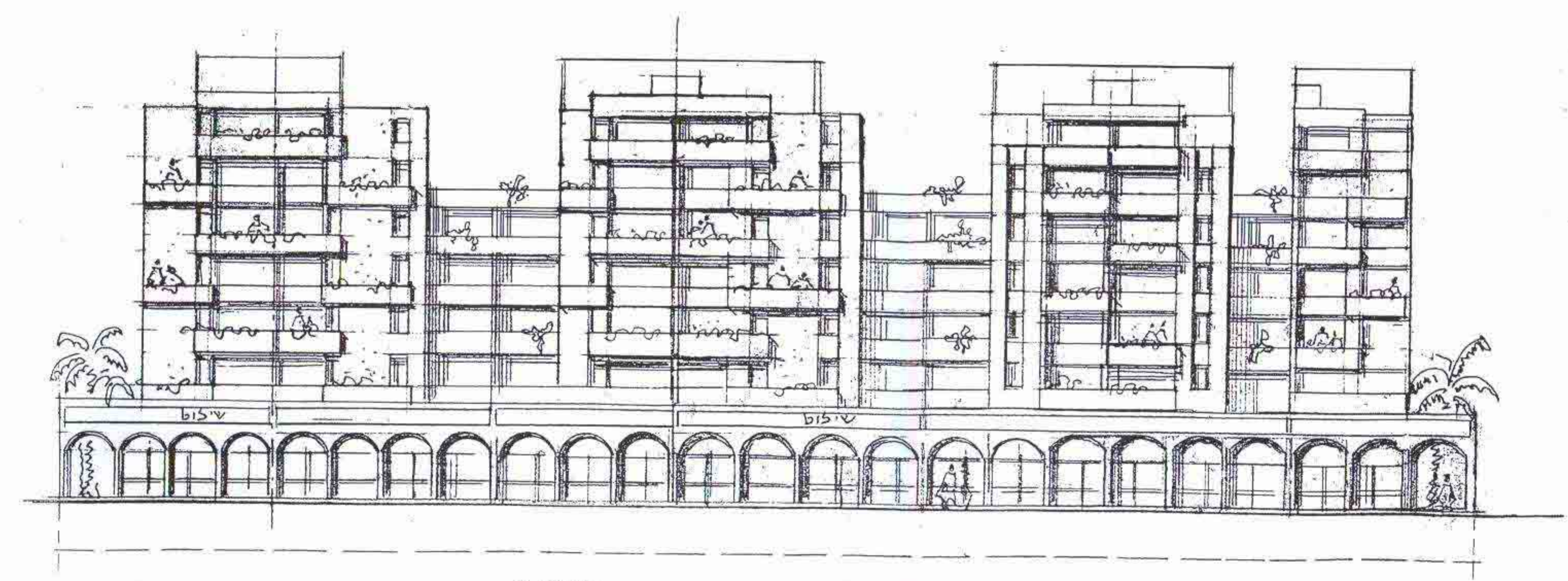
חזית לרחוב ויצמן ק.מ. 1:250
