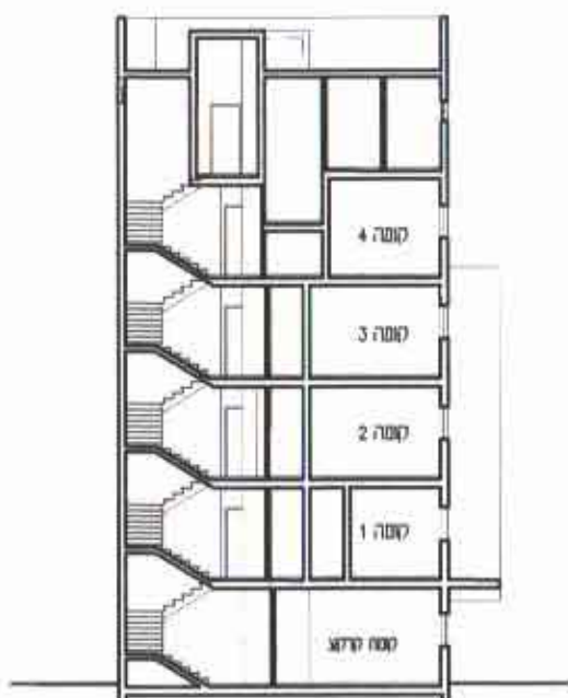
חתך א'-א'
