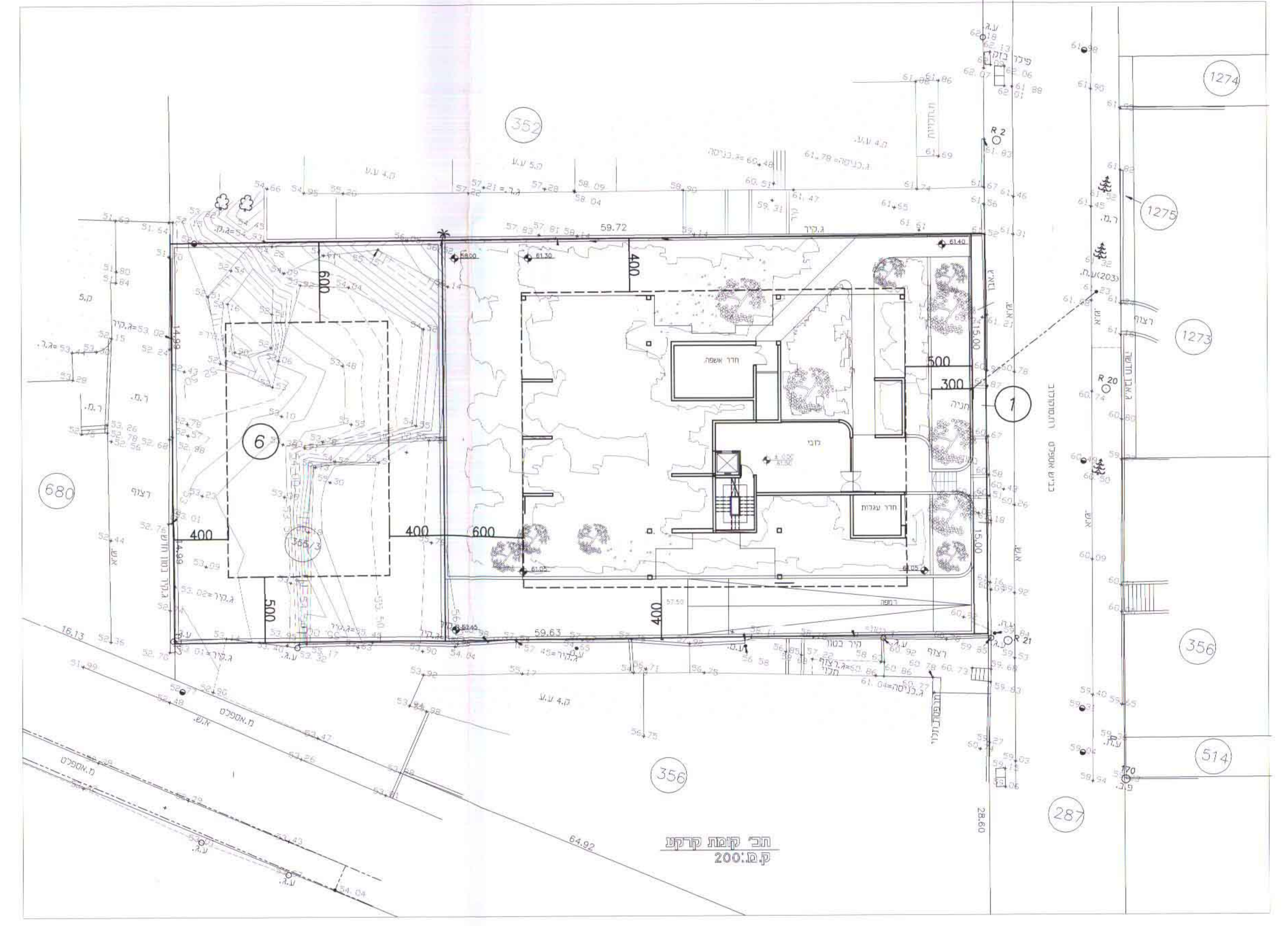
תוכנית קומת מרתף 200:מ.ק
