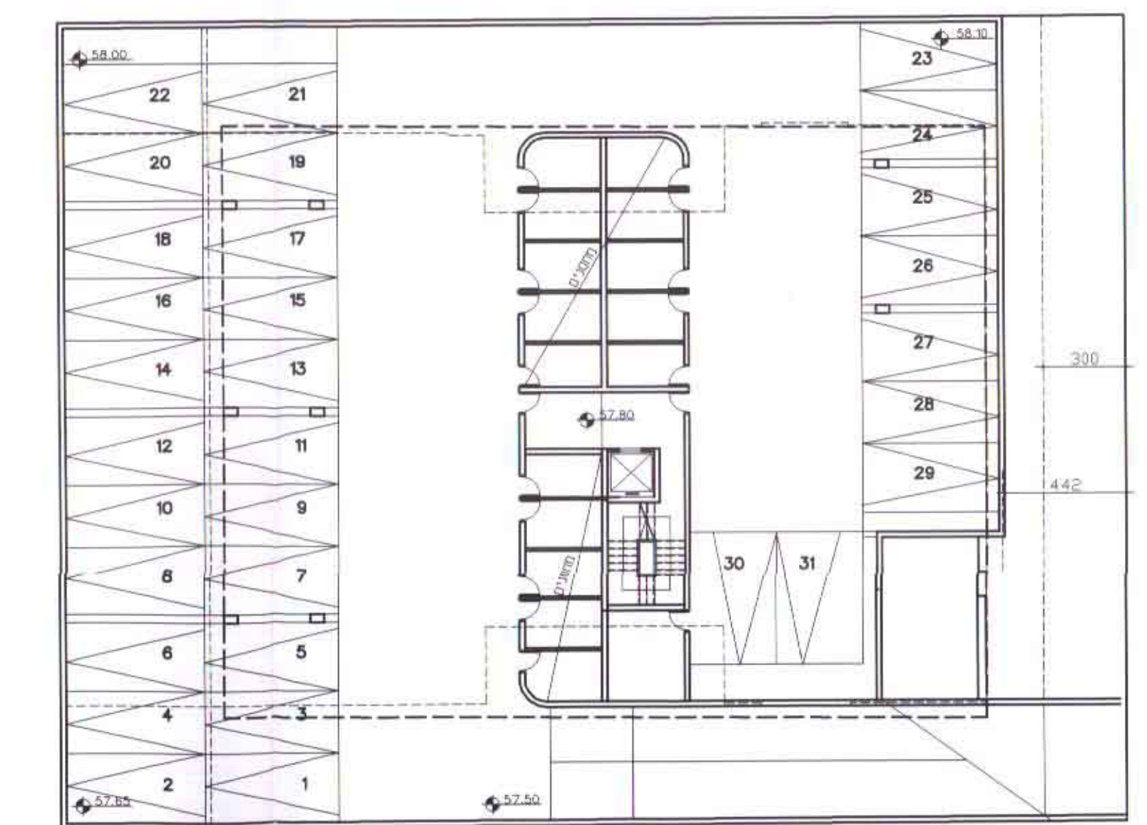
תוכנית קומת מרתף 200:מ.ק
