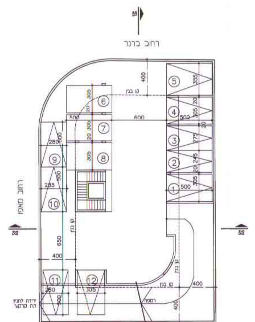
תכנית חניון תת קרקעי (עקרוני) קנה מידה 1:250
