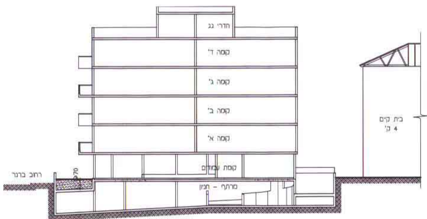
חתך עקרוני ב-ב קנה מידה 1:250
