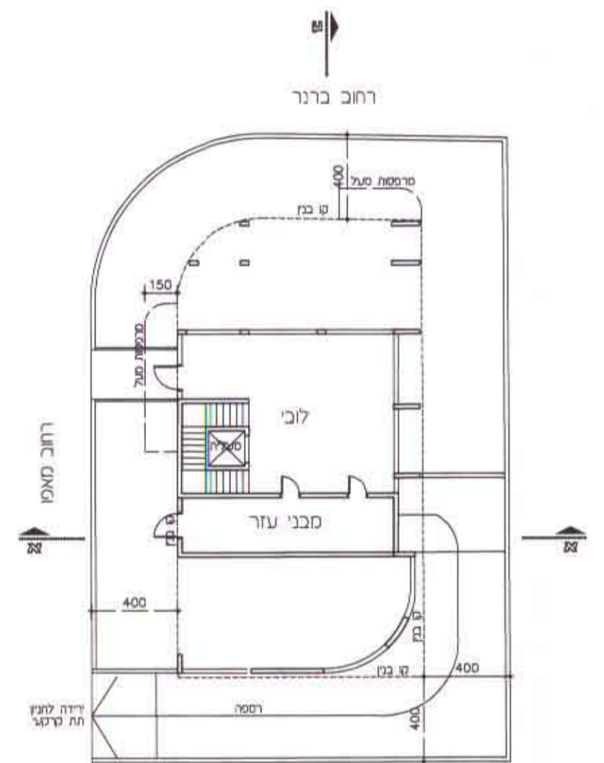
תכנית קומת קרקע (עקרוני) קנה מידה 1:250
