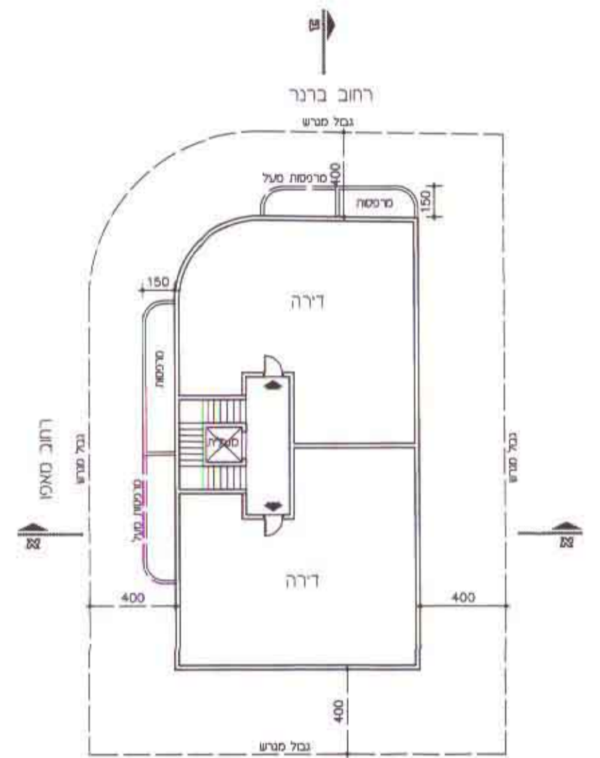
תכנית קומה טיפוסית (עקרוני) קנה מידה 1:250
