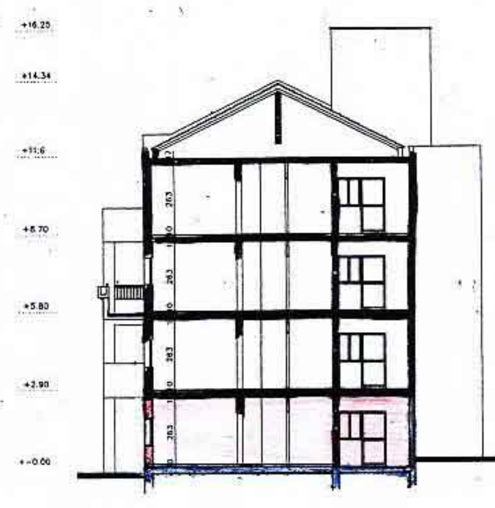
חתך - RA טיפוס 8 קנ"מ 1:200
