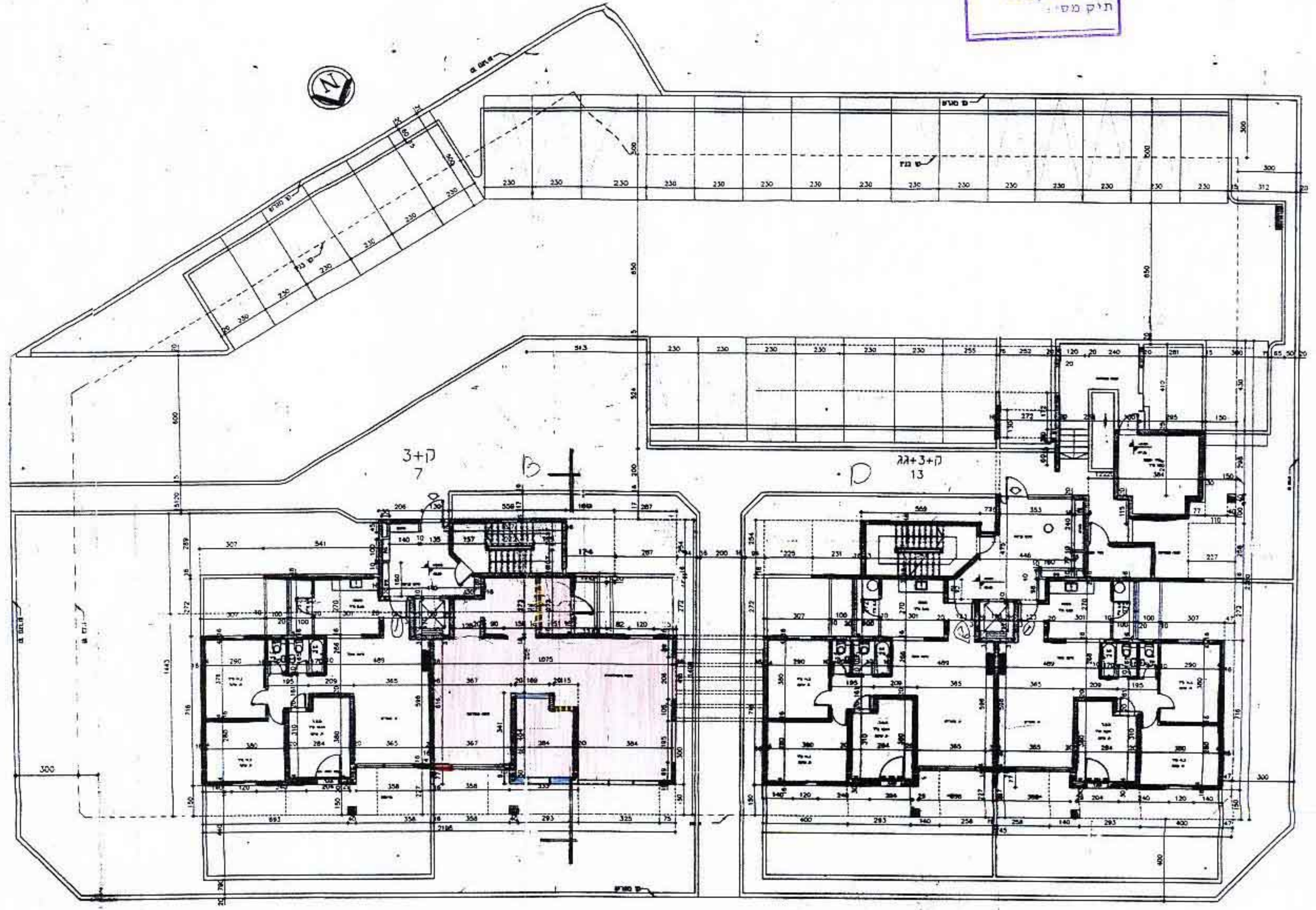
תכנית קומת הקרקע - מפלס +0.00 - קנ"מ 1:200 תכנית קומת הקרקע - מפלס +0.00 - קנ"מ 1:200
