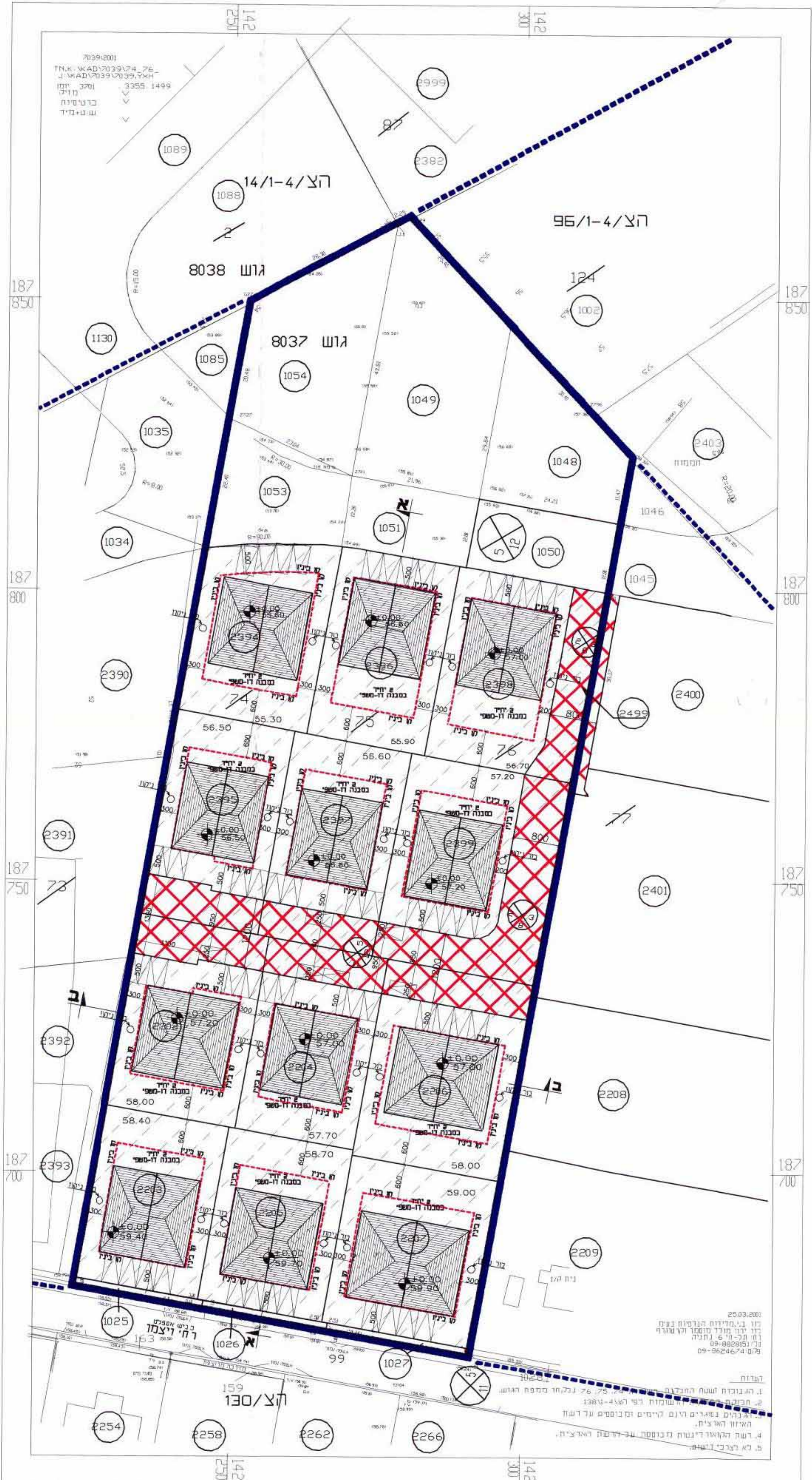
תוכנית בנייה מנחה עפ"י הצ/4-1/138 ג' קנ"מ 1 : 500
