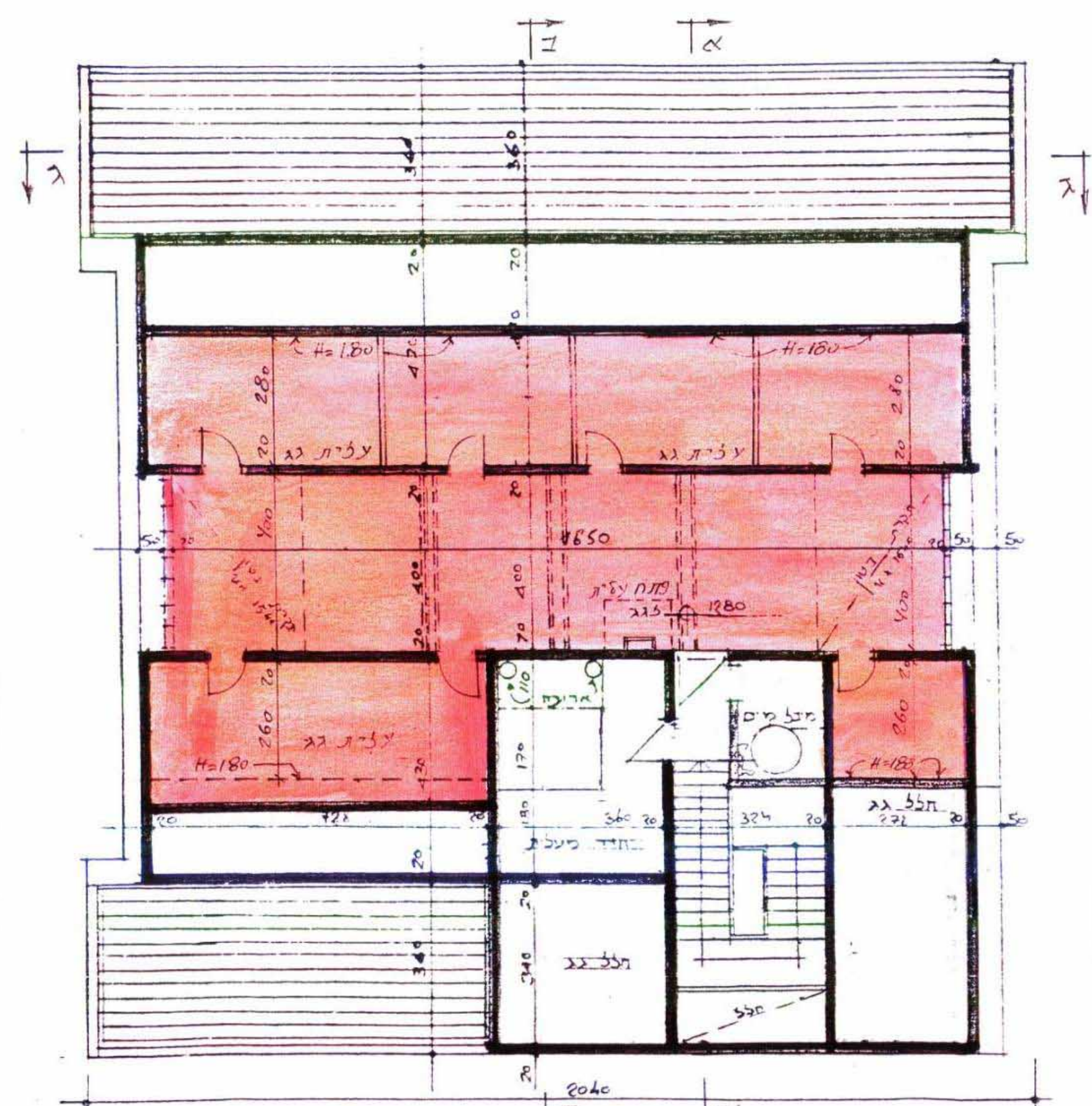
תכנית חלל-גג ק.מ. 1:100
