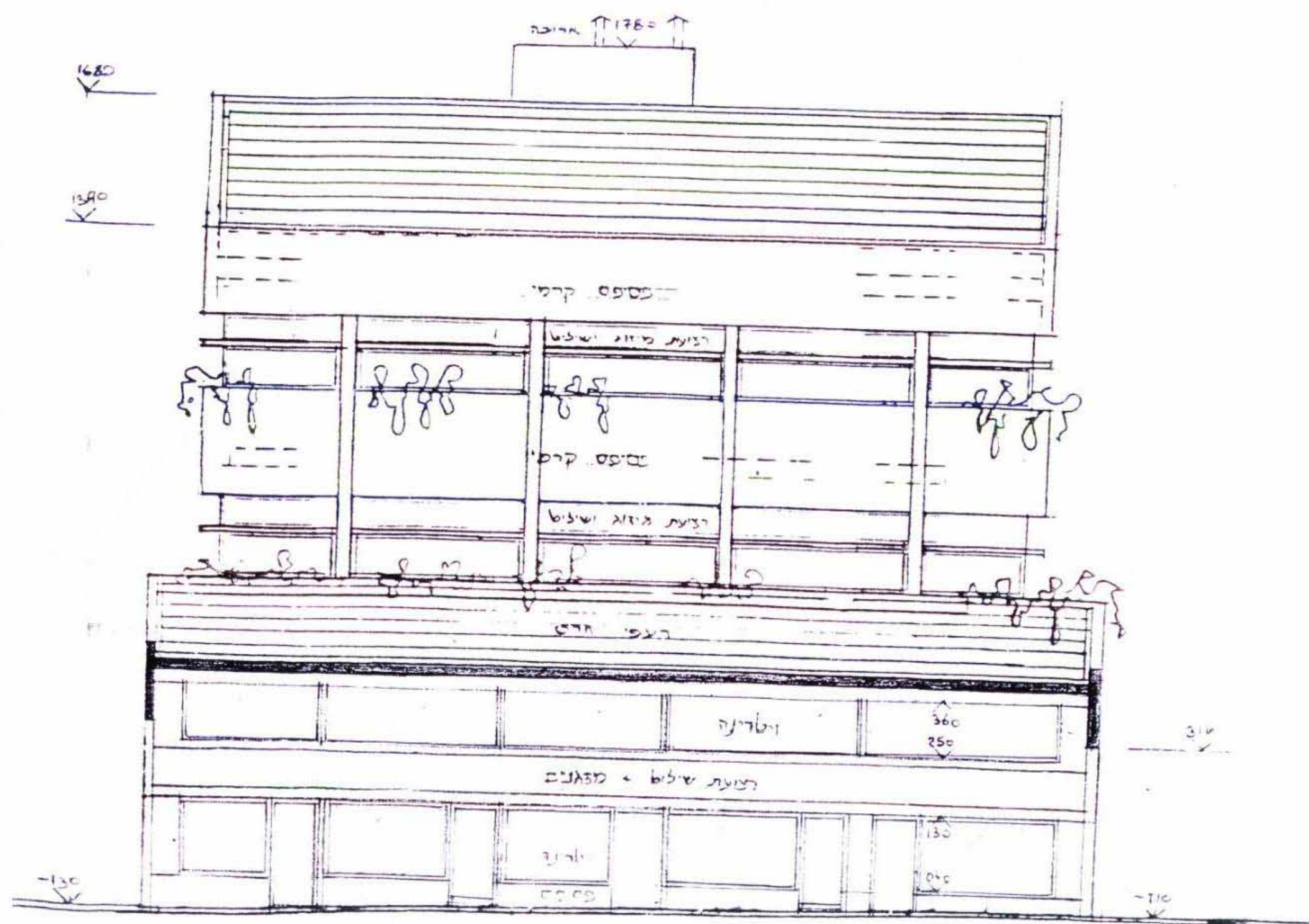
חתך ג-ג ק.מ. 1:100 חזית חנויות
