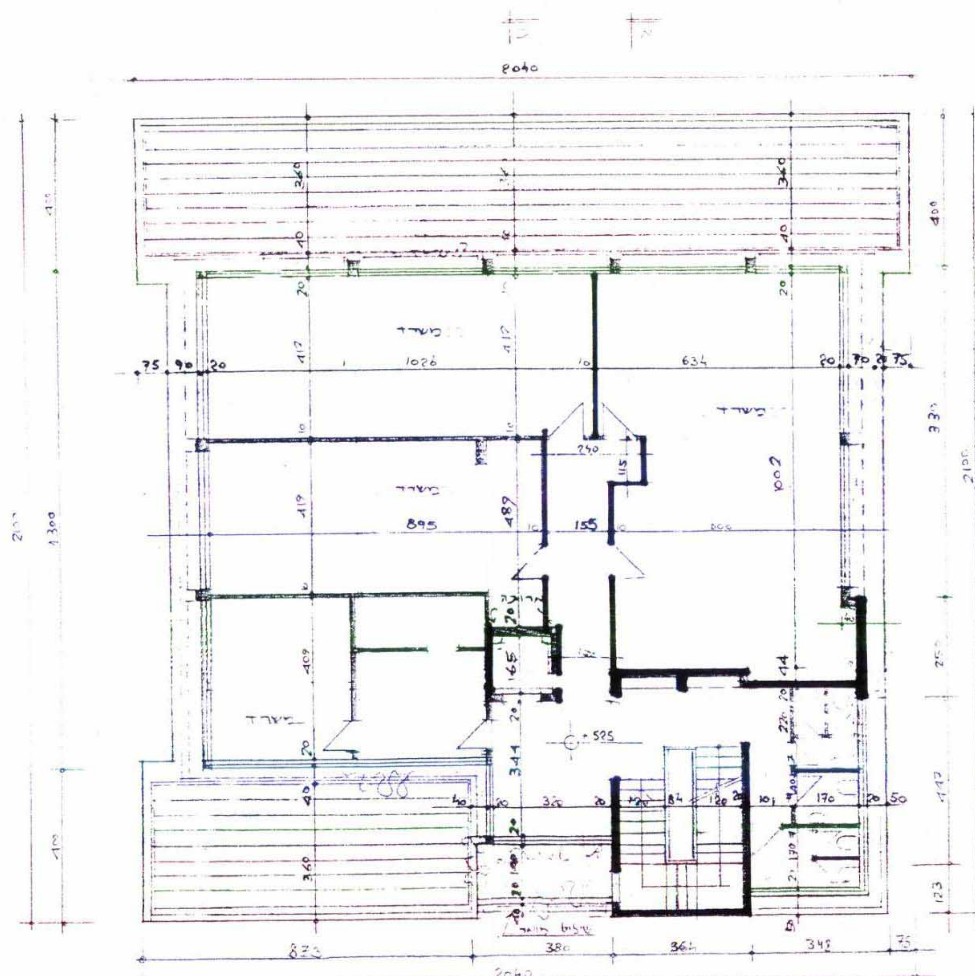
תכנית קומה א' - משרדים ק.מ. 1:100
