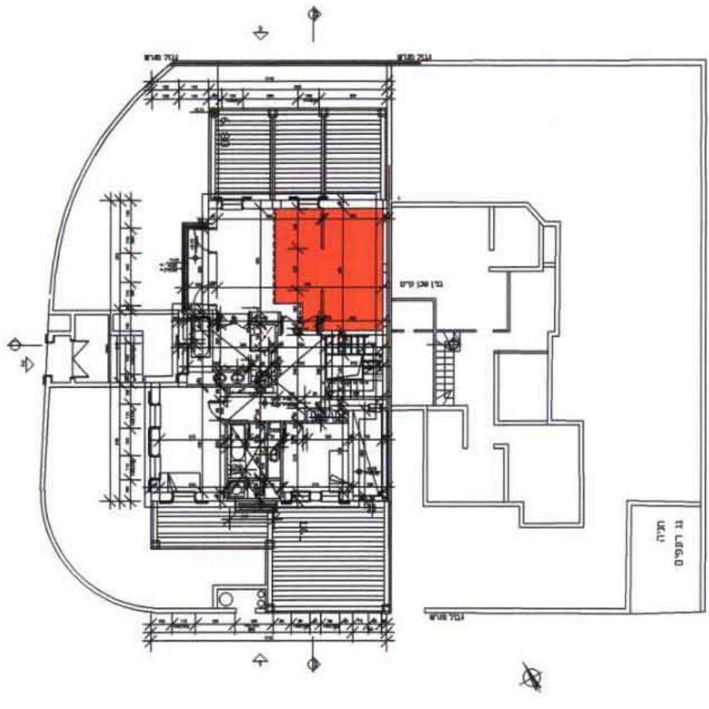
תוכנית קומה א' קנ"מ 1:250
