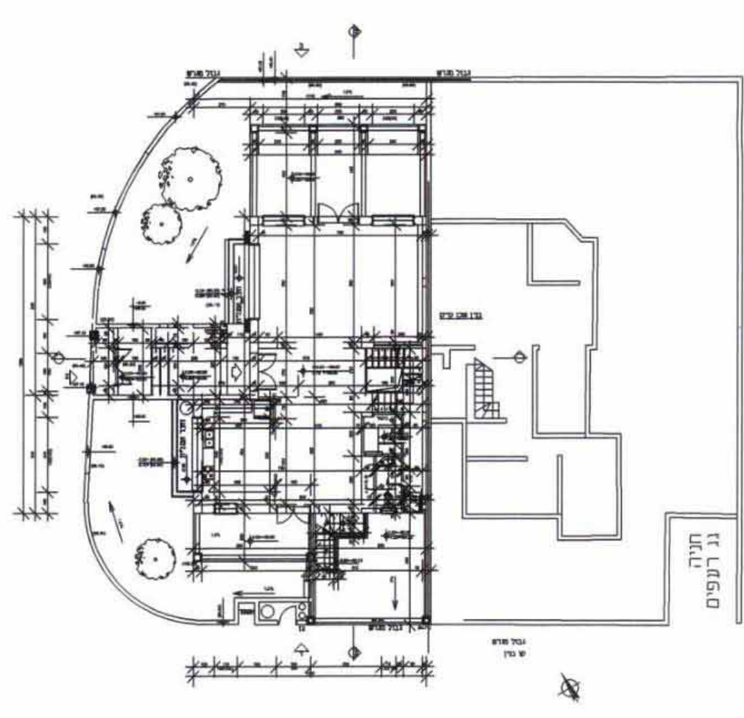
תוכנית ק. קרקע קנ"מ 1:250
