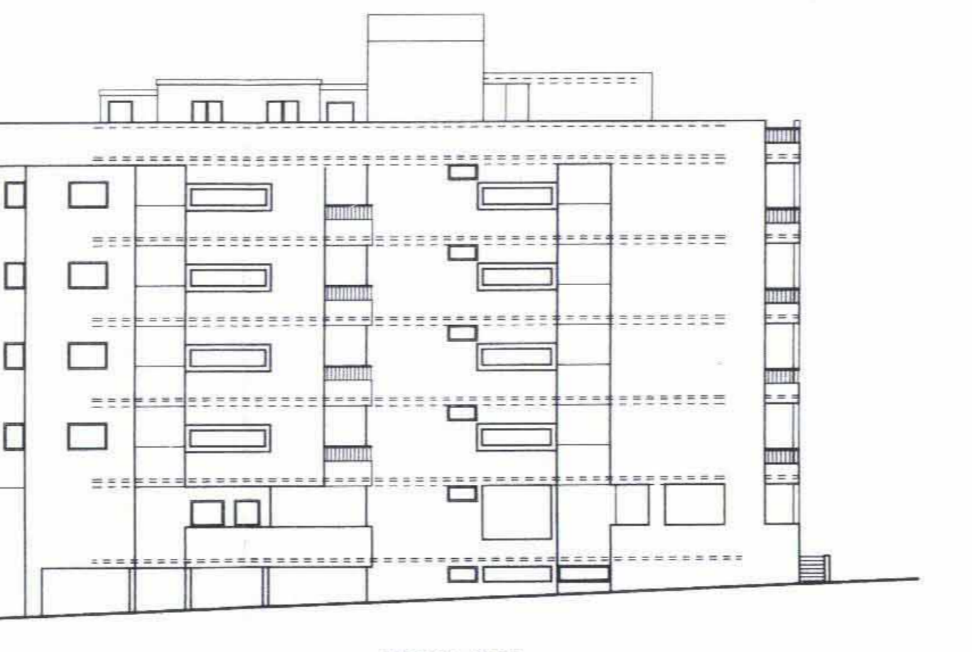
חזית צפנית 1 : 200
