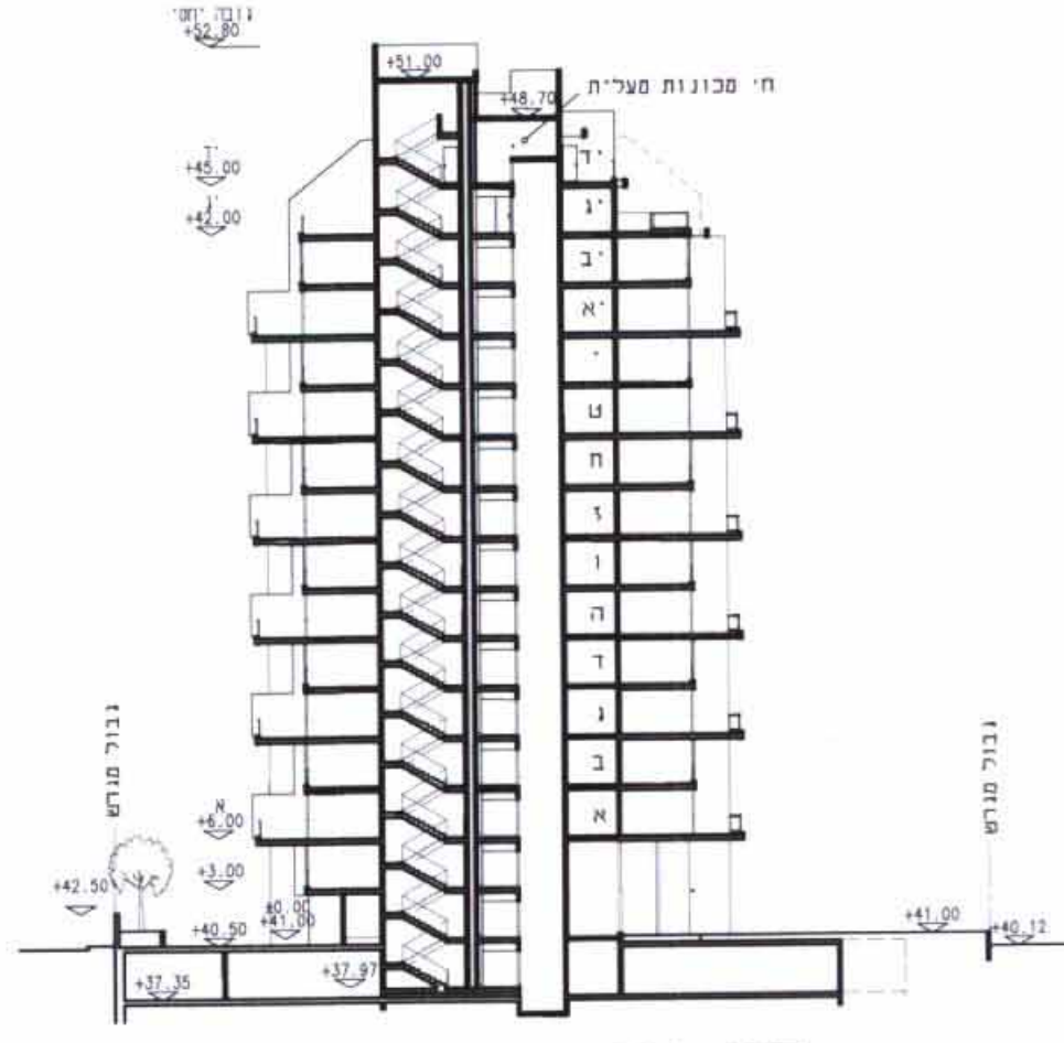
חתך 1:500
