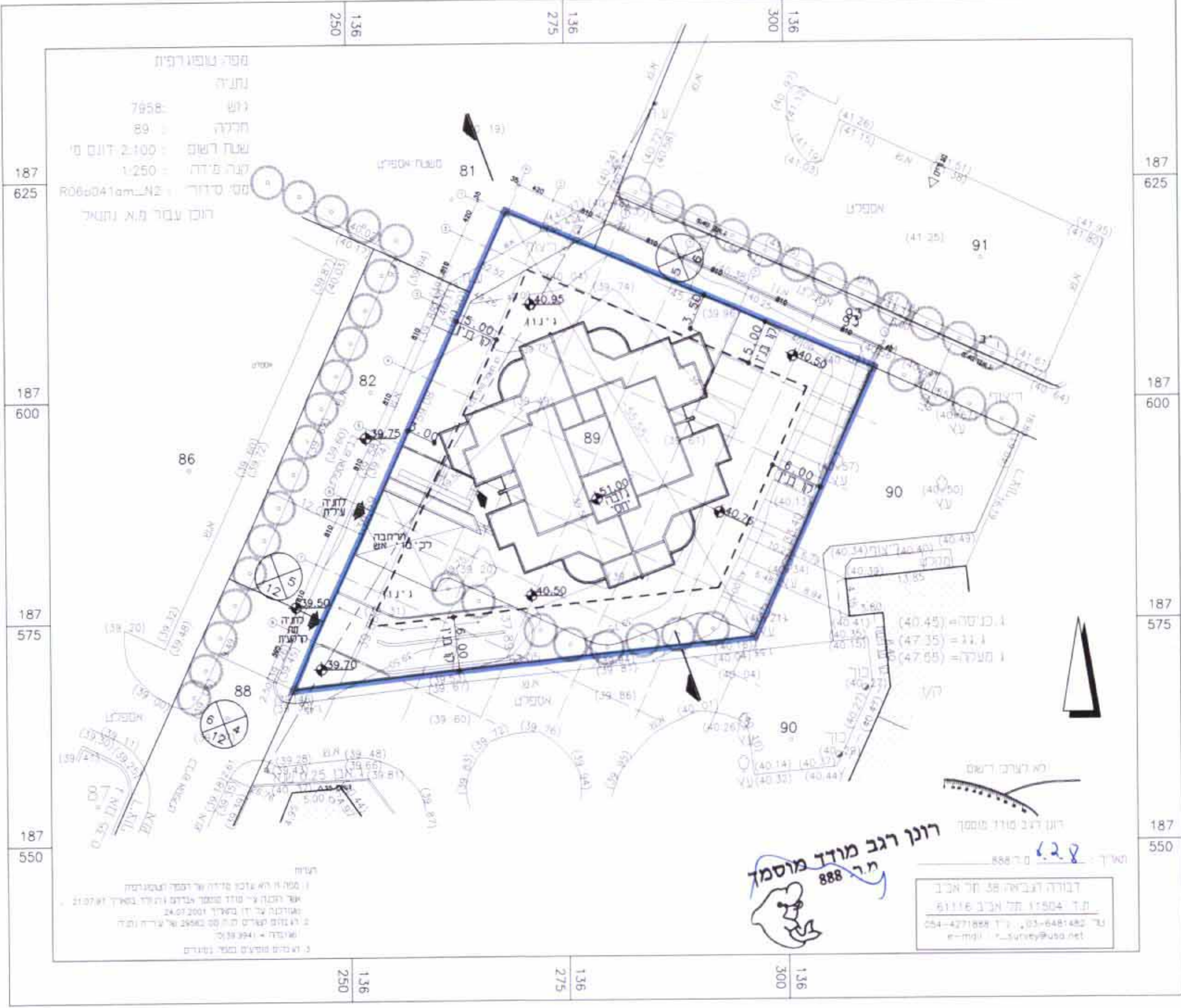
תכנית 1:500
