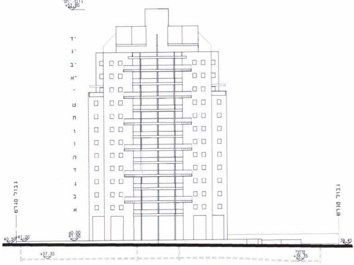
חזית צפון מערב קיים 1:500
