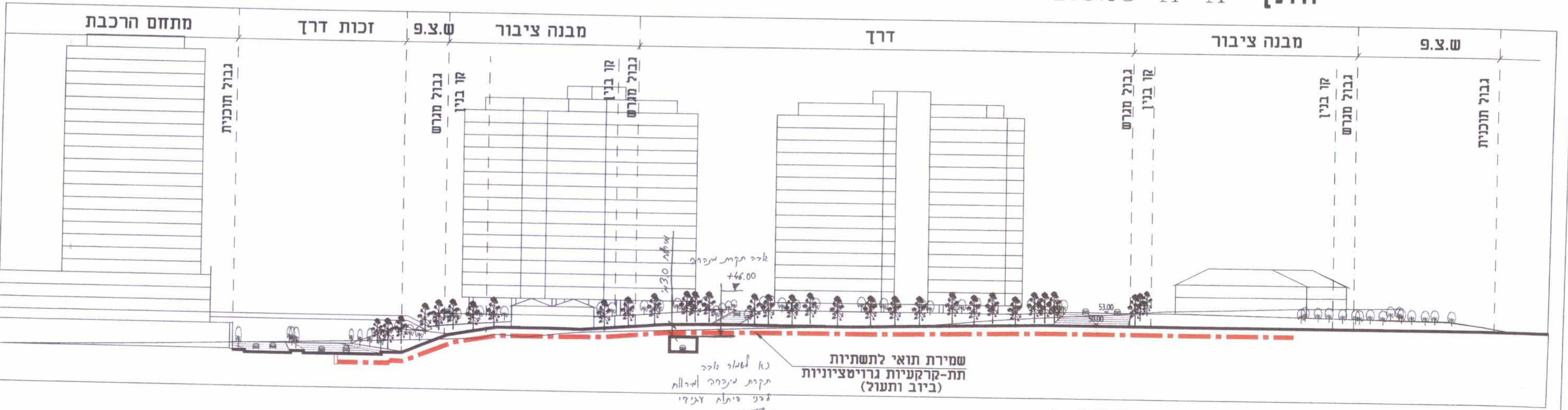
חתך 1:625 B-B
