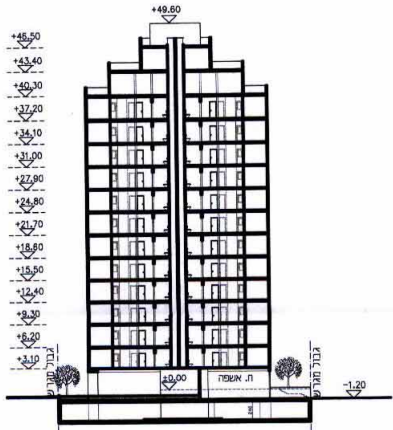
חתך עקרוני א-א ק.מ. 500 : 1
