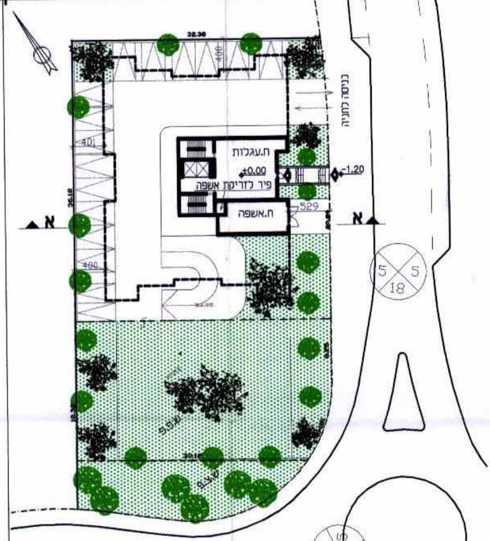
תכנית קומת קרקע ק.מ. 500 : 1
